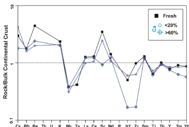
شکل ۲۰ تغییرات عناصر فرعی و برخی عناصر خاکی کمیاب بهنجار شده به پوسته‌ی قاره‌ای [۳۲] در نمونه‌های دگرسانی کربناتی در توده‌ی هورنبلند موزونیت پورفیری.
