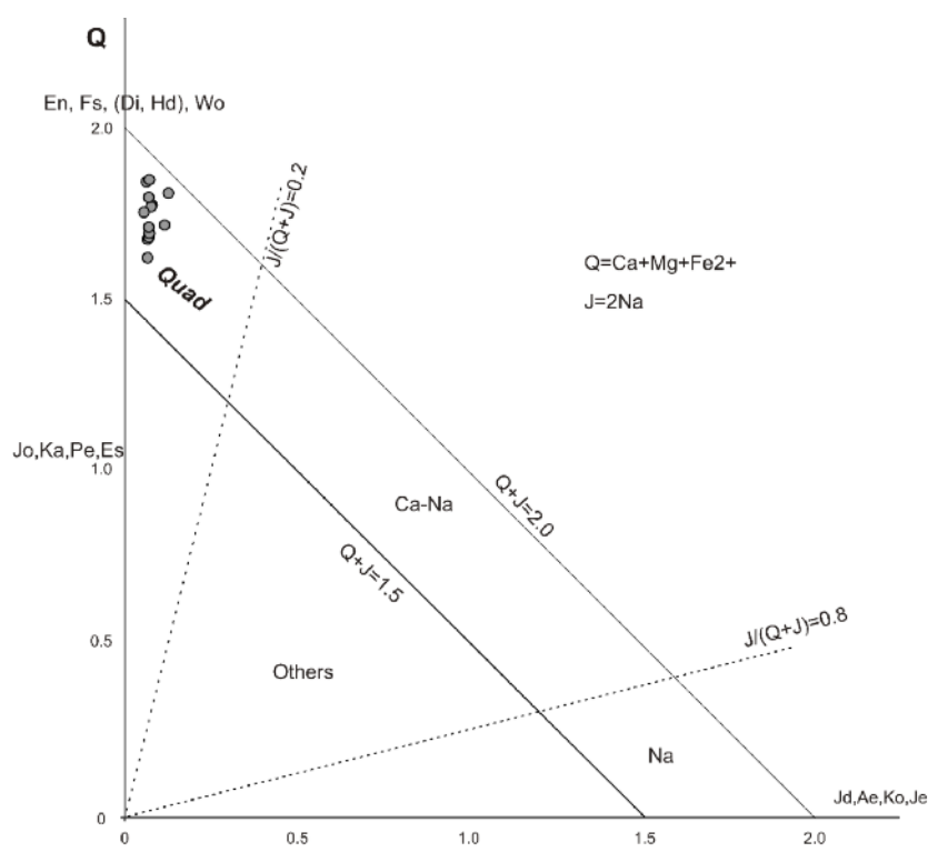
شکل ۶ کلینوپیروکسن‌های مورد بررسی در نمودار Q-J در گستره‌ی کلینوپیروکسن‌های کلسیم-منیزیم-آهن‌دار قرار می‌گیرند [۹].
