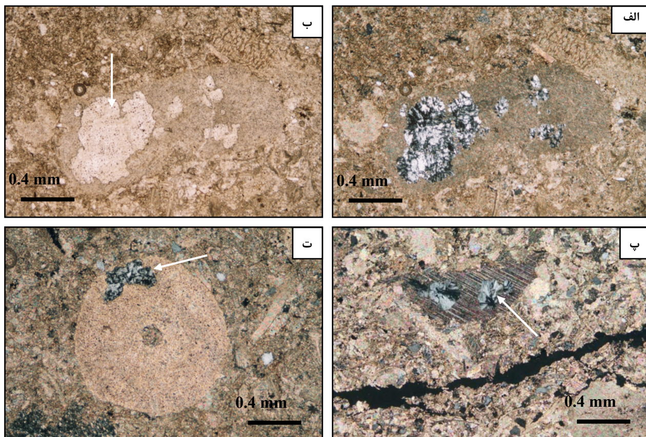
شکل ۳ الف) سیلیسی شدن بلورهای منفرد اکینودرم (XPL) ب) تصویر الف در PPL که بلور منفرد اکینودرم با حفره پر شده به وسیله سیلیس در آن بهتر تشخیص داده می‌شود. پ) خرده اکینودرم که در سطوح ضعیف رخ آن کوارتز کلسدونی جانشین شده است (XPL). ت) سیلیسی شدن به شکل کوارتز دانه‌ای در خرده اکینودرم (XPL).
