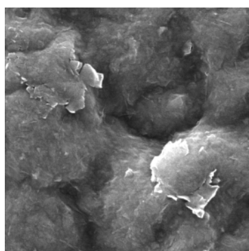
شکل ۶ تصویر میکروسکوپ الکترونی پویشی شکل ۷ تصویر میکروسکوپ الکترونی پویشی شکل ۸ تصویر میکروسکوپ الکترونی پویشی نمونه رسی بنتونیت با بزرگنمایی ۱۲۰۰۰ نمونه نانورس کلوزایت \text{Na}^+ با بزرگنمایی ۱۲۰۰۰ برابر نمونه رسی (SLB) با بزرگنمایی ۱۲۰۰۰ برابر
