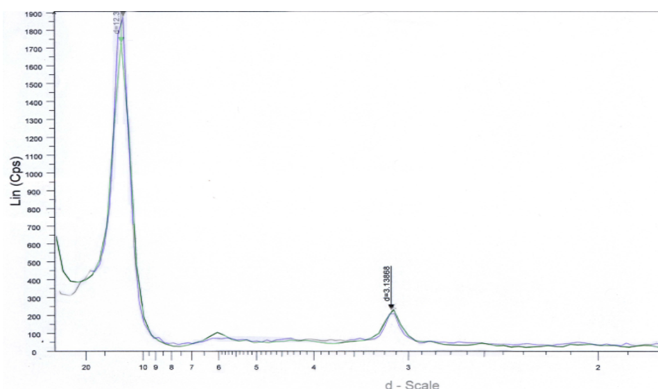
شکل ۴ مقایسه‌ی منحنی پراش پرتو ایکس نمونه‌ی مونت‌موریلونیت SLB و نانو مونت‌موریلونیت کلوزایت \text{Na}^+ .
