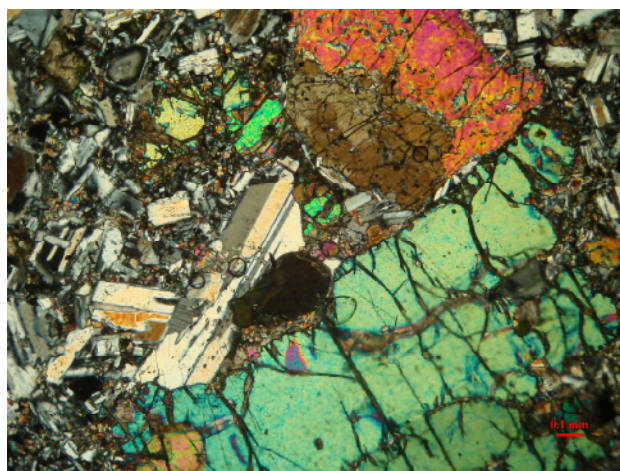
شکل ۲ اولیوین بازالت منطقه داماش حاوی بلورهای اولیوین، پیروکسن و پلاژیوکلاز (با آنالیزور XPL)
