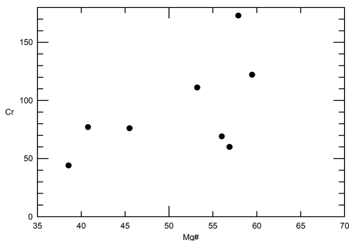
شکل ۷ نمودار تغییرات \text{Cr} نسبت به عدد منیزیم برای سنگ‌های داماش.
