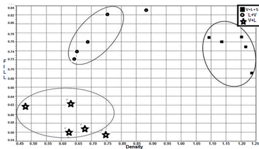
شکل ۱۰ موقعیت چگالی میانبارهای شاری نسبت به پرشدگی آن. میانبارهای شاری نوع A ( L + V + S ) با درجه‌ی پرشدگی و چگالی بالا، میانبارهای شاری نوع B ( V + L ) با چگالی پائین و درجه‌ی پرشدگی کم، میانبارهای شاری نوع C ( L + V ) با شوری متوسط و درجه پرشدگی بالا
