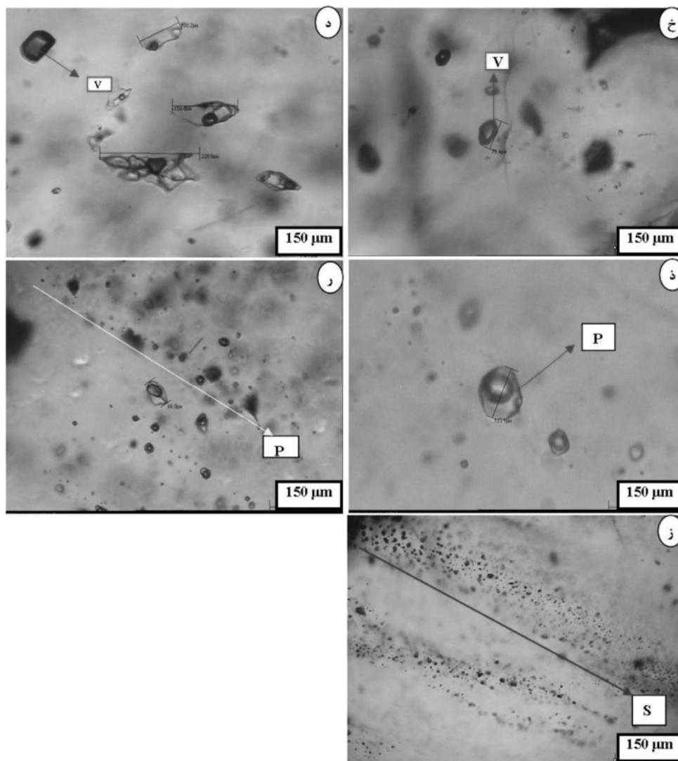
شکل ۹ خ، د، میانبارهای شاری تک فاز گاز د، میانبارهای شاری اولیه ر، تصاویر میانبارهای شاری ثانویه ی کاذب ز، تصاویر میانبارهای شاری ثانویه.
