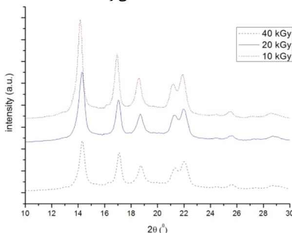
شکل ۱۲ طیف پرتو ایکس پلی پروپیلن تابش دهی شده با دزهای متفاوت.
