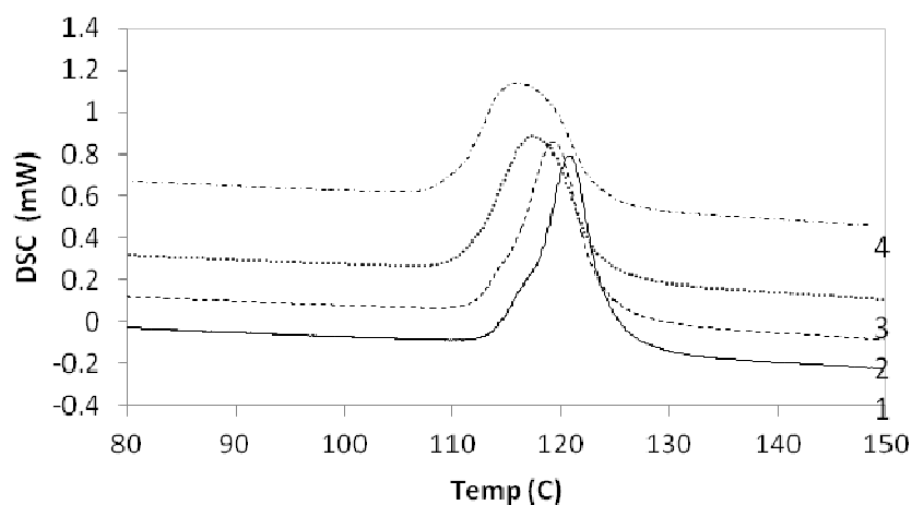
شکل ۷ منحنی DSC پلی پروپیلن سرد شده در (۱): هوا، (۲) کاست، (۳): تحت فشار و (۴): ازلت.
