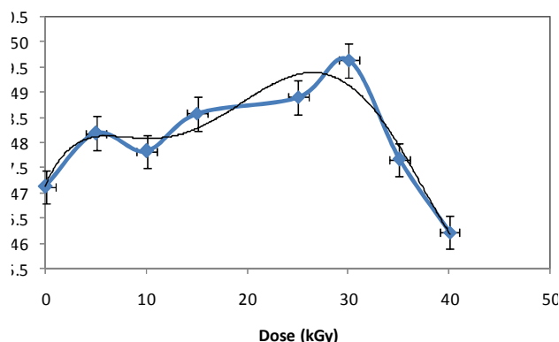
شکل ۸ تغییرات درصد بلورینگی نمونه های پلی پروپیلین تابش دهی شده با دزهای مختلف به روش DSC.
