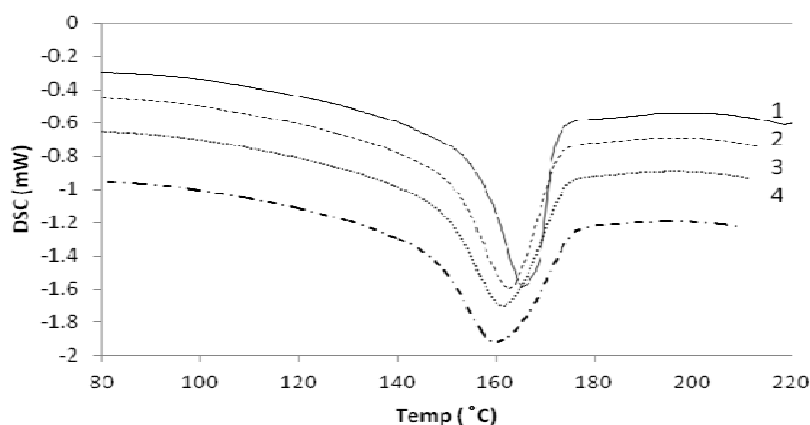
شکل ۶ منحنی DSC پلی پروپیلن ذوب شده در (۱): هوا، (۲) کاست، (۳): تحت فشار و (۴): ازلت.
