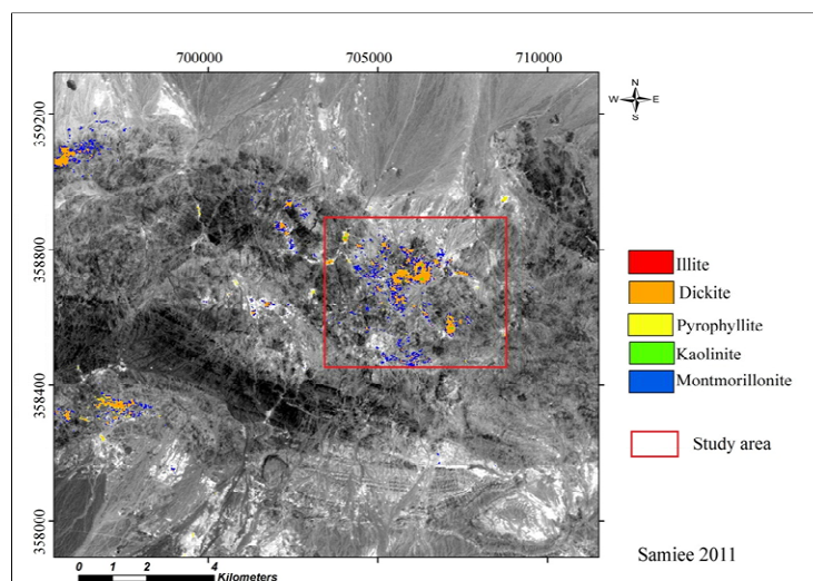
شکل ۲ تصویر ماهواره‌ای آستر، که دگرسانی آرژلیک روی آن آشکارسازی شده است.
