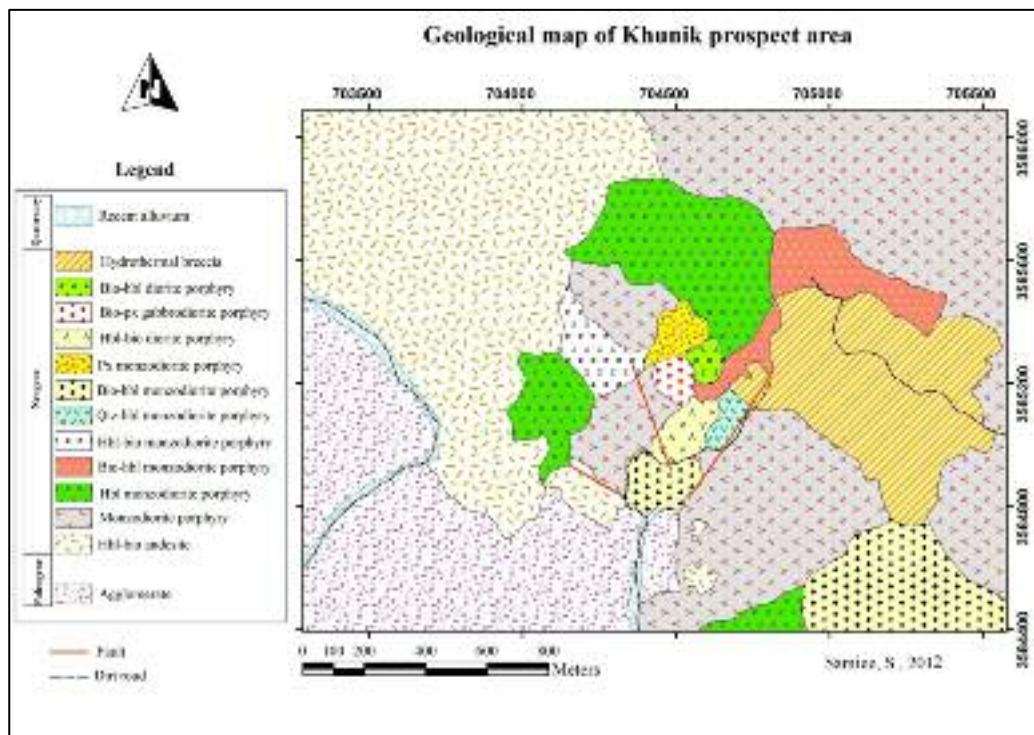
شکل ۵ نقشه زمین‌شناسی منطقه اکتشافی خونیک.
