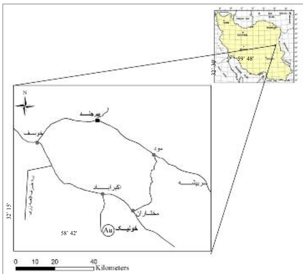
شکل ۱ موقعیت جغرافیایی و راه‌های دسترسی به منطقه مورد مطالعه.
