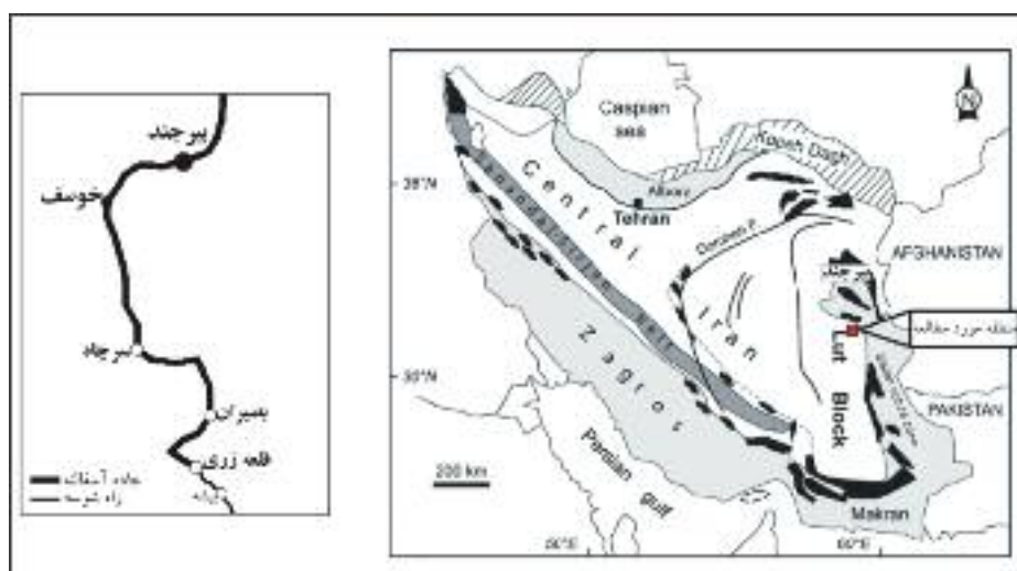
شکل ۱. نقشه تقسیمات ساختاری ایران [۱] با تغییرات و موقعیت منطقه‌ی مورد بررسی، به همراه نقشه راه‌های دسترسی.
