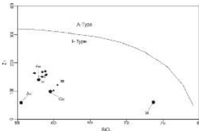
شکل ۱۲ نمودار تغییرات Zr نسبت به \text{SiO}_2 [۳۹] نمونه‌های مورد بررسی (علائم مانند شکل ۵)، به همراه موقعیت میانگین نفوذی‌های همراه با اسکارن‌های مختلف بریتیش کلمبیا [۳۱].
