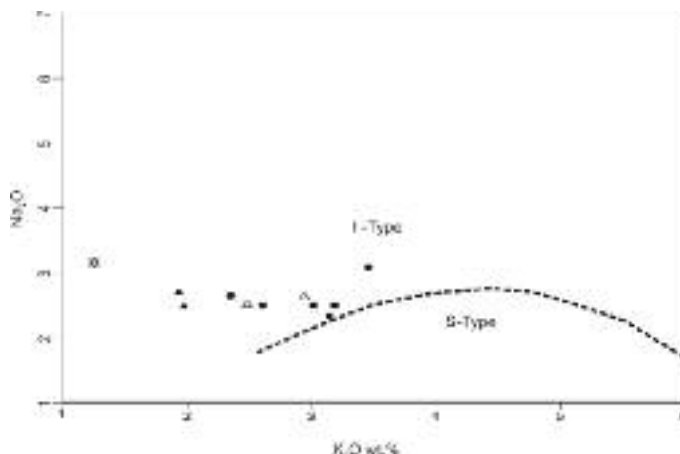
شکل ۱۱ نمودار تغییرات \text{Na}_2\text{O} نسبت به \text{K}_2\text{O} که در آن محدوده گرانیت‌های I و S از یکدیگر جدا شده‌اند [۳۷] (علائم مانند شکل ۵).
