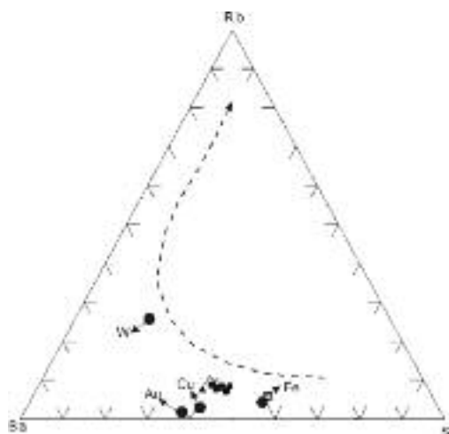
شکل ۱۰ مثلث Rb-Ba-Sr [۲۰] و میانگین توده‌های نفوذی همراه با اسکارن‌های مختلف بریتیش کلمبیا [۳۱] (دوایر تو پر) به همراه نمونه‌های گرانیتوئیدی منطقه‌ی مورد بررسی (علائم مانند شکل ۵)، (پیکان خط چین راستای جدایش را نشان می‌دهد).
