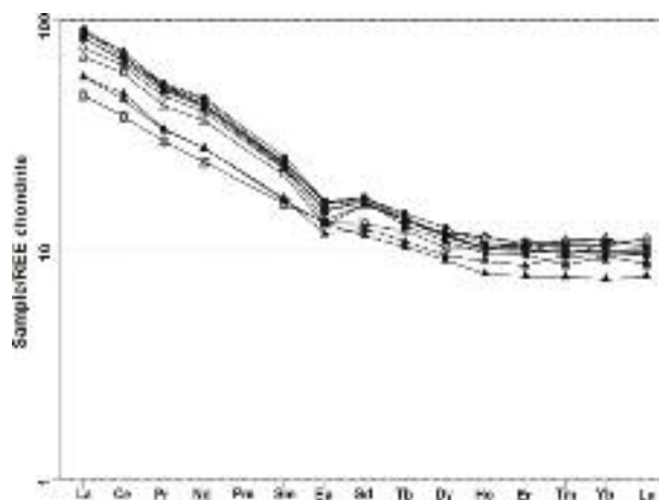
شکل ۱۴ نمودار عناصر نادر خاکی بهنجار شده با کندریت [۴۷] برای سنگ‌های گرانیتوئیدی بیشه (علائم مانند شکل ۵).
