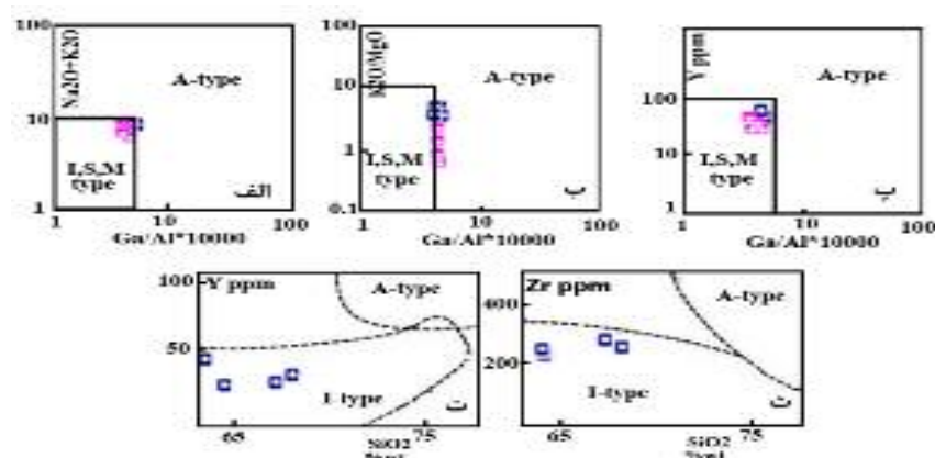
شکل ۷ نمودارهای جدایش گرانیتوئیدهای A، S و M از [۱۹] و موقعیت نفوذی‌های منطقه‌ی پیرکوه روی آنها: الف) درصد وزنی \text{Na}_2\text{O}+\text{K}_2\text{O} نسبت به \text{Ga}/\text{Al} \times 10000 ، ب) \text{K}_2\text{O}/\text{MgO} نسبت به \text{Ga}/\text{Al} \times 10000 ، پ) \text{Y} برحسب ppm نسبت به \text{Ga}/\text{Al} \times 10000 ، و نیز نمودارهای عناصر HFS نسبت به \text{SiO}_2 [۲۰] (ت) \text{Y} در مقابل \text{SiO}_2 ، ث) \text{Zr} در مقابل \text{SiO}_2 (مفهوم علائم همانند شکل ۴-ب).
