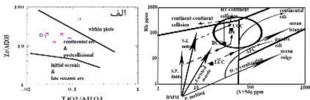
شکل ۹ (الف) داده‌های وابسته به سنگ‌های نفوذی منطقه‌ی پیرکوه روی نمودار TiO_2/Al_2O_3-Zr/Al_2O_3 [۱۵] (مفهوم علائم همانند شکل ۴-ب) و (ب) مسیر فرآیندهای مؤثر روی خاستگاه گرانیت‌ها و نقطه‌ای که یک گرانیت نمونه با خاستگاه گوشته‌ای که ممکن است در اثر این فرآیند به آن برسد. همچنین ترکیب پوسته‌ی قاره‌ای بالائی (UCC) و ترکیب کلی آن (BCC)، و نیز مسیری که ذوب بخشی ترکیب کلی پوسته‌ی قاره‌ای تغییر یافته به وسیله‌ی شارها می‌تواند در طول راندگی در یک جایگاه همزمان با برخورد طی کند نمایش داده شده‌اند (SZ منطقه فرورانش) [۱۷].
