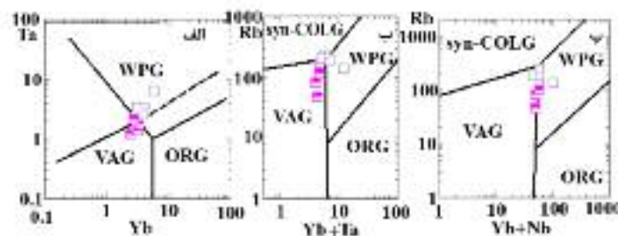
شکل ۸ داده‌های وابسته به سنگ‌های نفوذی منطقه‌ی پیرکوه روی نمودار جدایشی گرانیتوئیدها بر اساس، الف) \text{Ta}-\text{Yb} [۱۷] خطوط شکسته در نمودارهای بالا مرز VAG و ORG وابسته به پشته‌های غیرعادی را نشان می‌دهند. ب) \text{Rb}-(\text{Yb}+\text{Ta}) و پ) \text{Rb}-(\text{Y}+\text{Nb}) [۱۷] (مفهوم علائم همانند شکل ۴-ب).
