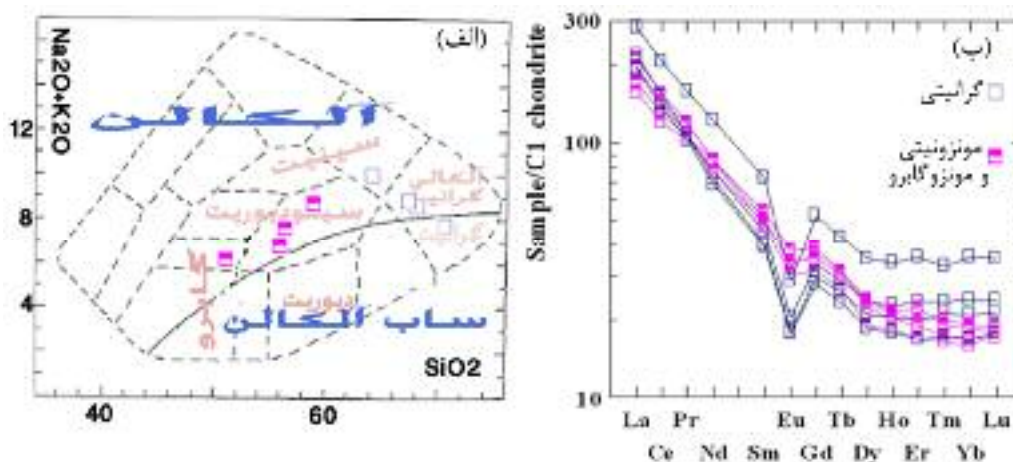
شکل ۴ الف) رده‌بندی سنگ‌های نفوذی بر اساس نمودار TAS [۹] که توسط [۱۰] برای سنگ‌های نفوذی تعمیم داده شده است. ب) الگوهای REE نمونه‌های آذرین نفوذی منطقه پیرکوه که به مقادیر کندریتی ارائه شده توسط [۱۱] به‌نچار شده‌اند.
