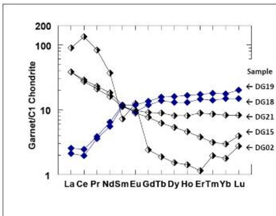
شکل ۷ الگوی رفتاری عناصر کمیاب خاکی در گارنت‌های اسکارن دره‌ی زرشک. علائم اختصاری: DG02، DG15 و DG21 گارنت‌های با ترکیب آن‌را دیتی، DG18 و DG19 گارنت‌های با ترکیب گراسولاری.
