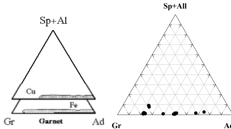
شکل ۹ نمودار توزیع ترکیب تجزیه‌های ریزکائوئیدی الکترونی گارنت‌های اسکارن دره‌ی زرشک و مقایسه آن‌ها با ترکیب گارنت‌های انواع نهشته‌های اسکارنی [۱۱،۱۰]. علائم اختصاری: Gr: گراسولار، Ad: آندرادیت، Sp: اسپسارتین، Al: آلماندن.
