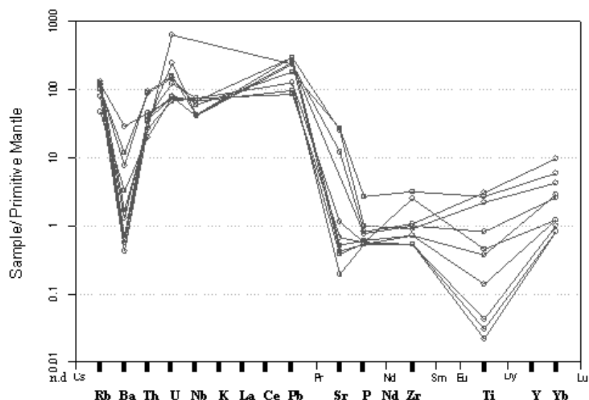
نمودار ۱. نمودارهای همبستگی اکسید عناصر فرعی (بر حسب PPM) در کانسار کرومیت کوهی.
