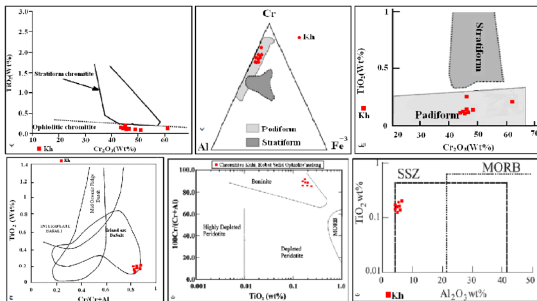
شکل ۵. الف) نمودار TiO_2 نسبت به Cr_2O_3 [۱۸]. ب) نمودار مثلثی Cr, Fe^{3+}, Al (پ) نمودار TiO_2 نسبت به Cr_2O_3 [۲۸، ۱۹]. ت) تعیین محیط زمین‌ساختی و وزن کرومیت‌های محدوده کوهی براساس دیاگرام مقدار TiO_2 نسبت به Cr/(Cr + Al) [۲۹]. ث) نمودار Cr/(Cr + Al) نسبت به TiO_2 [۲۹]. ج) نمودار Al_2O_3 نسبت به TiO_2 [۲۴].
