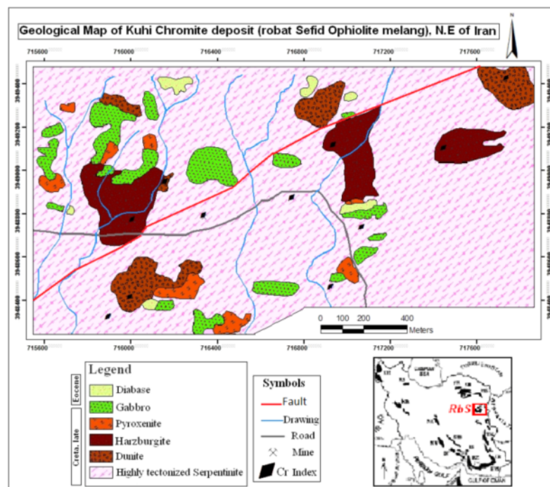
شکل ۱ نقشه‌ی زمین شناسی با مقیاس ۱:۱۰۰۰۰ کرومیت کوهی (واقع در افیولیت ملانژ شمال تربت حیدریه).
