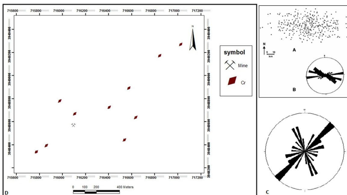
شکل ۴ (الف) توزیع شاخص‌های کرومیت و (ب) Rosdigram ترسیم شده گسل‌های افیولیت رباطسفید. (پ) روند گسل‌ها و درزهای گستره‌ی مورد بررسی نقش شده در نمودار رزیدیاگرام با نرم افزار StereoNet. (ت) موقعیت شاخص‌های کرومیت کوهی.
