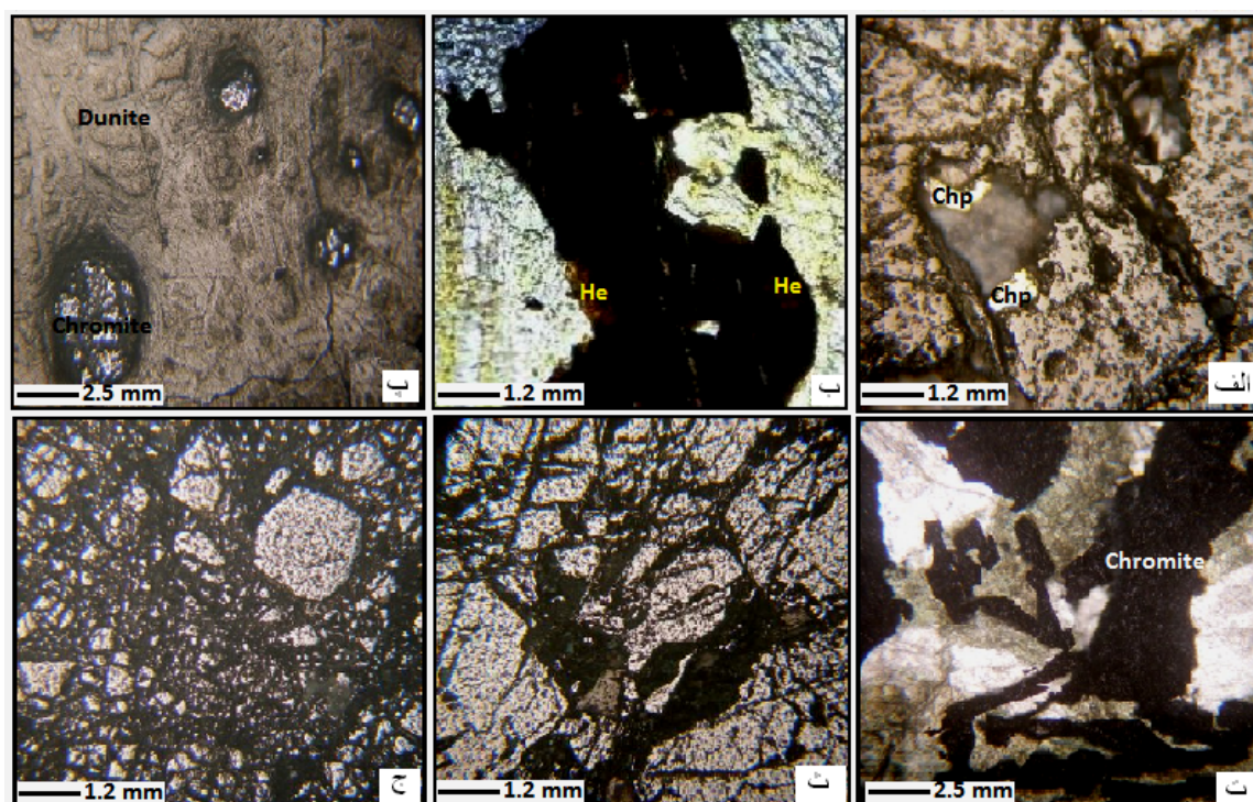
شکل ۳ الف) کرومیت با بافت توده‌ای به همراه کانی‌سازی کالکوپیریت (Chp) در (PPL) بازتابی. ب) برون‌رست فاز هماتیت از کرومیت در حاشیه دانه کرومیت در XPL عبوری. پ) کرومیت با بافت‌افشان (بافت اولیه)، تک بلورهای کرومیت در زمینه‌ای از سیلیکات‌ها (الیون) در (PPL) بازتابی. ت) بافت کششی (بافت ثانویه)، در اثر افزایش حجم ناشی از سرپانتینی شدن سیلیکات‌های دربرگیرنده در (PPL) عبوری. ث) بافت برشی (بافت ثانویه) بلورهای کاملاً خردشده کرومیت که به‌وسیله سیلیکات‌ها به هم متصلند در (PPL) انعکاسی. ج) بافت کاتاکلاستی (بافت ثانویه) خردشدگی و شکستگی دانه‌های کرومیت در (PPL) انعکاسی.
