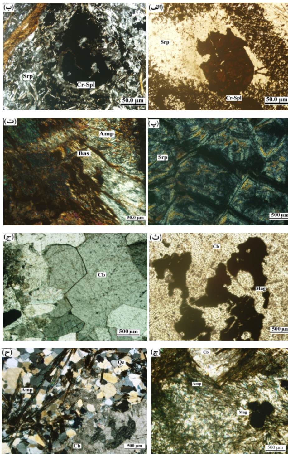
شکل ۳ تصاویر میکروسکوپی سرپانتینیت‌ها و لیستونیتهای دگرگون شده موجود در افیولیت بیاض.
