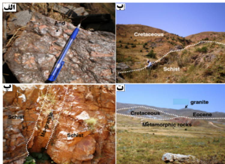
شکل ۲ (الف) بلورهای آندالوزیت به اندازه ۴-۵ cm در آندالوزیت شیت. (ب) قرارگیری ماسه سنگ‌های سرخ کرتاسه روی واحدهای دگرگون (دید به سمت غرب). (پ) دایک موسکوویت گرانیتی در داخل شیست‌ها (دید به سمت غرب) (ت) توده نفوذی گرانیت-گرانودیوریت داخل واحدهای ائوسن (دید به سمت شمال شرقی).
