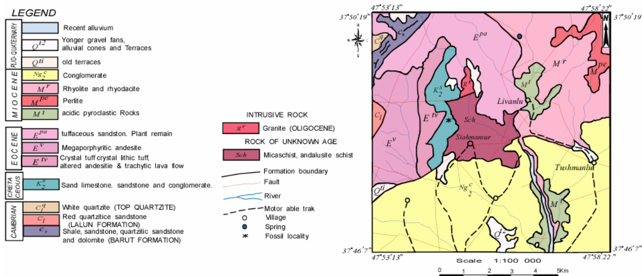
شکل ۱. نقشه‌ی زمین‌شناسی منطقه با اقتباس از نقشه‌ی زمین‌شناسی ۱/۱۰۰۰۰۰ سراب [۴].
