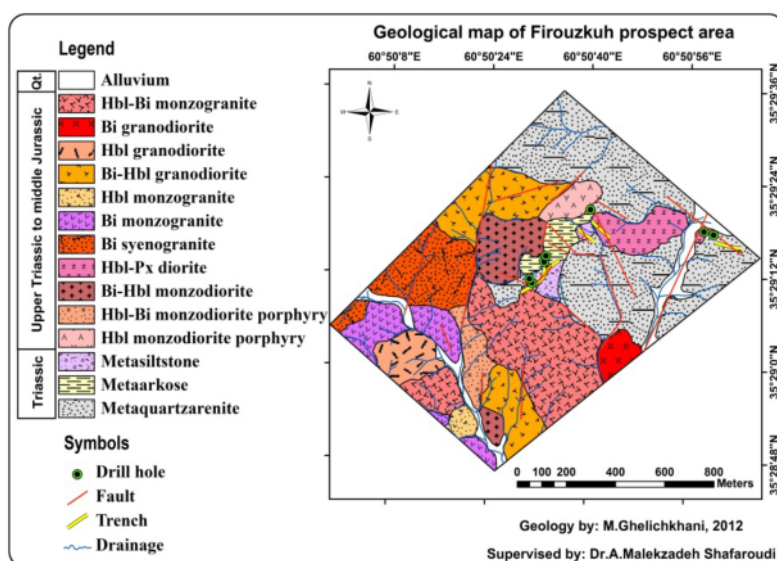
شکل ۲ نقشه زمین‌شناسی منطقه‌ی پی‌جوی فیروزکوه همراه با موقعیت گمانه‌ها و ترانشه‌های حفر شده.
