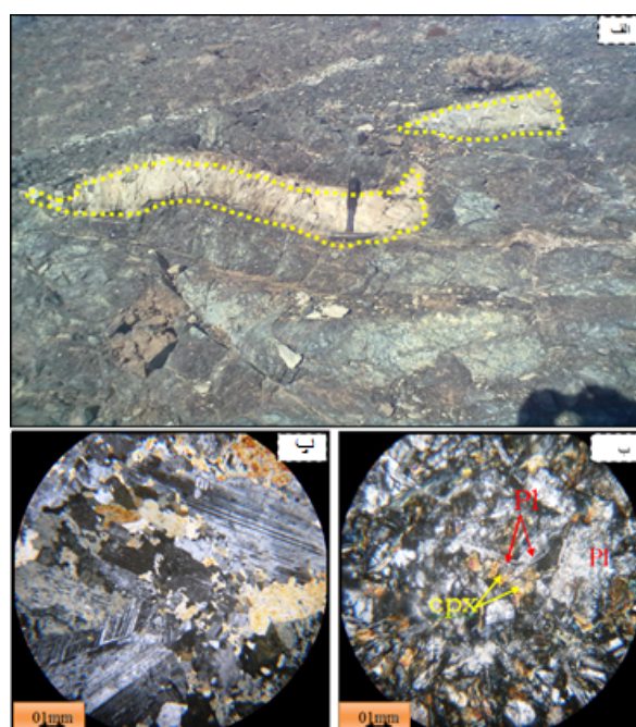
شکل ۲ الف) نفوذ دلریتها در سنگ‌های الترامافیک منطقه ب) نمایش بافت افتیک و ساب‌افتیک در دولریت‌های منطقه مورد بررسی پ) نمایش بافت پوئی‌کلریتیک همراه با ماکل پلی‌سنتتیک در پلاژیوکلاز. (PL) پلاژیوکلاز، (CPX) کلینوپیروکسن.
