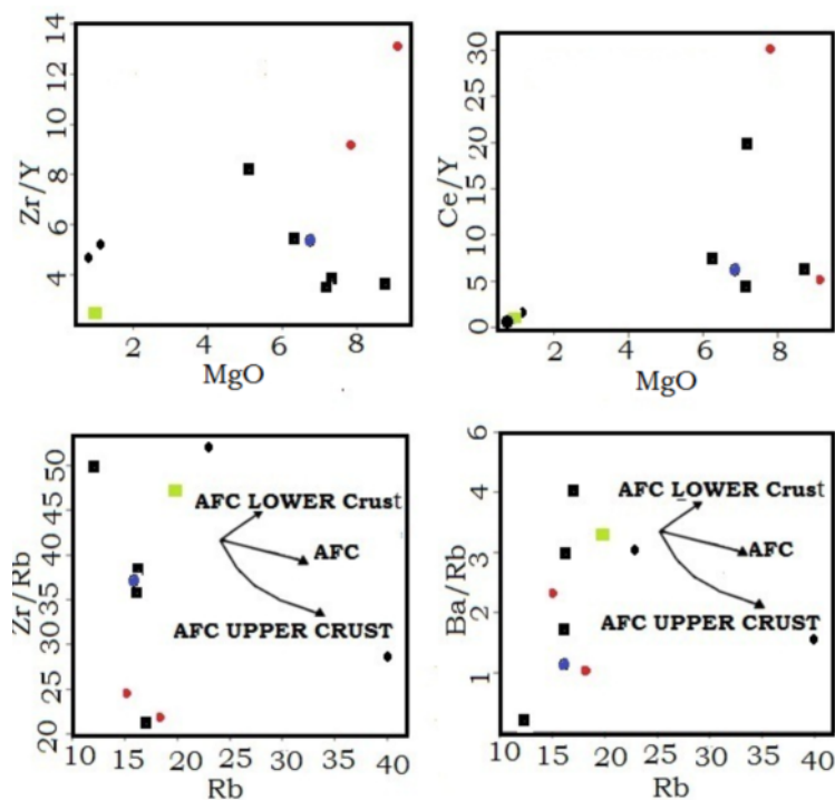
شکل ۸. نمودار Mg در برابر Zr/Y و Ce/Y [۱۱] و نمودار Rb نسبت به Zr/Rb و Ba/Rb [۱۲] جهت بررسی نقش فرآیند آلیش پوسته‌ای در سنگ‌های منطقه‌ی مورد بررسی.
