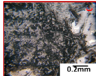
شکل ۶ الف، حضور پیریت در گرانیت‌های شمال منطقه. ب، حضور کالکوپیریت در منطقه‌ی گسله جنوب منطقه. پ، تبدیل کالکوپیریت به کوولیت. ت، تبدیل پیریت به گوئیت با بافت باقیمانده و آتول. ث، رگچه‌ی هماتیت و گوئیت. ج، رگچه‌ی آزوریت در منطقه‌ی گسله جنوب‌شرق منطقه.
