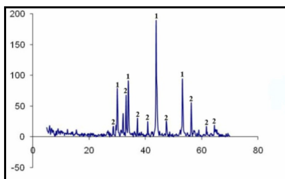
شکل ۱۴ الگوی پراش پرتو X، مربوط به پیرویت و پیریت موجود در اسکارن‌های منطقه‌ی مورد بررسی. ۱: پیرویت، ۲: پیریت.
