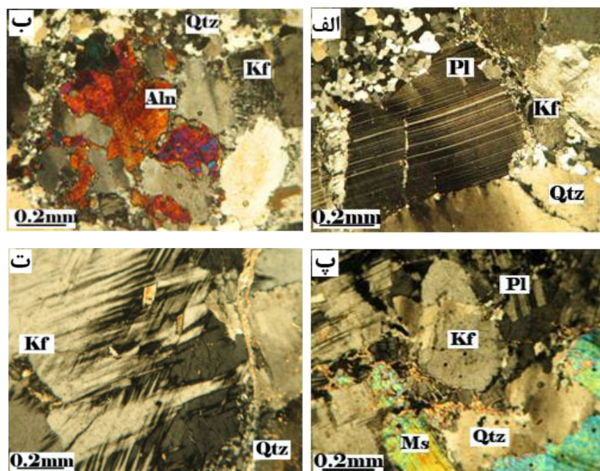
شکل ۳ تصاویر میکروسکوپی نمونه‌های پگماتیتهای منطقه در نور XPL. الف) گرانودیوریت پگماتیتهای با کوارتزهای ساب‌گرین شده و پلاژیوکلاز با ماکل‌های خمیده. ب) حضور آلانیت در پگماتیت‌های منطقه. پ) مونزودیوریت پگماتیتهای ت) ارتوکلاز دگرشکل شده حاوی ماکل تارتن (میکروکلین) در برخی قسمت‌های بلوره‌های آن. Pl: پلاژیوکلاز، Kf: فلدسپار پتاسیم، Qtz: کوارتز، Ms: موسکوویت، Aln: آلانیت.
