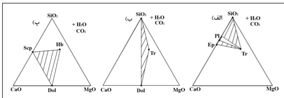
شکل ۱۶ نمودارهای ترکیب - پاراژنز [۲۹]، واکنش‌های صورت گرفته در اسکارن‌های منطقه‌ی ابراهیم عطار. Ep: اپیدوت، Dol: دولومیت، Sph: اسکاپولیت، Tr: ترمولیت کوارتز، Pl: پلاژیوکلاز، Hb: هورنبلند.
