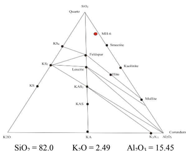
شکل ۱۰ سیستم ۳ تایی \text{SiO}_2 - \text{K}_2\text{O} - \text{Al}_2\text{O}_3 و ترکیب نمونه‌ی MH-6 [۱۴].
