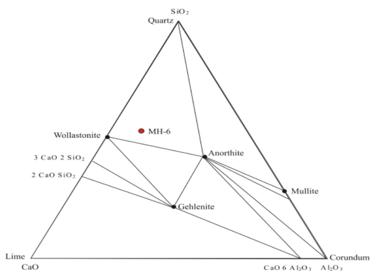
شکل ۸ سیستم ۳ تایی CaO-SiO_2-Al_2O_3 و ترکیب نمونه‌ی MH-6 [۱۴].
