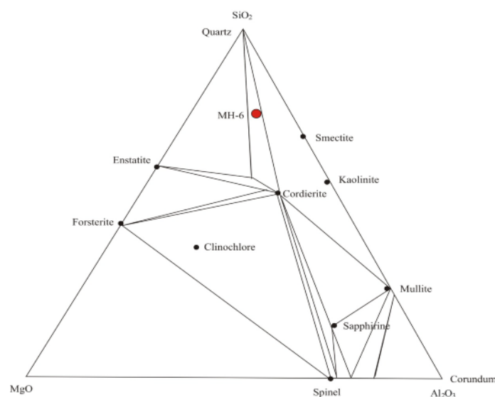
شکل ۹ سیستم ۳ تایی SiO_2-MgO-Al_2O_3 و موقعیت نمونه‌ی MH-6 [۱۴].
