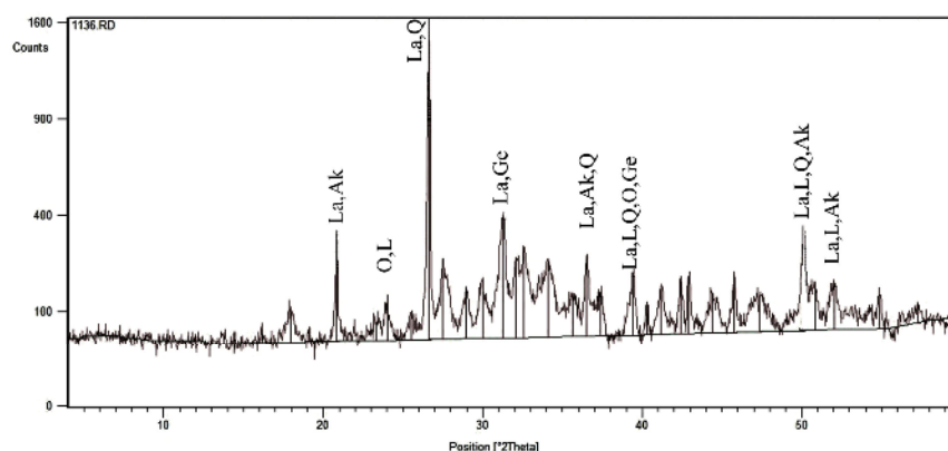
راهنما: Q: کوارتز-ژلنیت-اکرمانیت La: لارنیت-ژلنیت-اکرمانیت Ak: اورتوکلاز-ژلنیت-اکرمانیت Ge: اورتوکلاز-ژلنیت-اکرمانیت O: اورتوکلاز-ژلنیت-اکرمانیت شکل ۱۱ پراش نگاشت حاصل از آنالیز پراش پرتو ایکس (XRD)، نمونه‌ی آجر MH-6.
