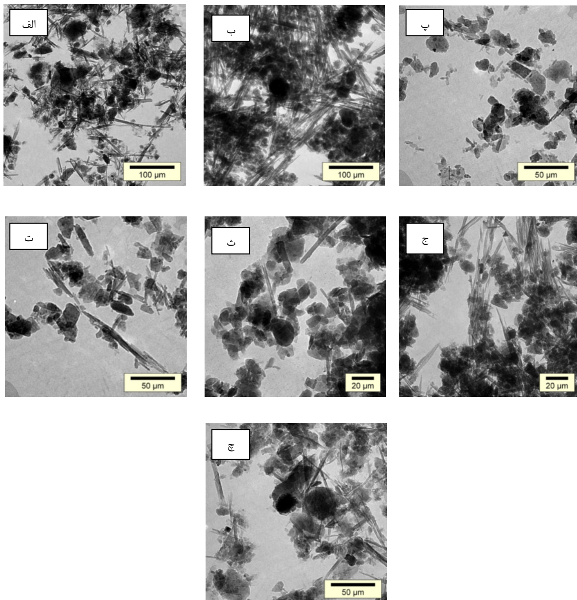
شکل ۴ ریزنگاشت میکروسکوپ الکترونی عبوری افق‌های By2 (الف) و Btmyz (ب) خاکرخ ۱، Az (پ) و Btmyz (ت) خاکرخ ۲، Az (ث)، By2 (ج) و C (ج) خاکرخ ۳ نشان دهنده بلورهای دسته جارویی و منفرد پالیگورسکیت
