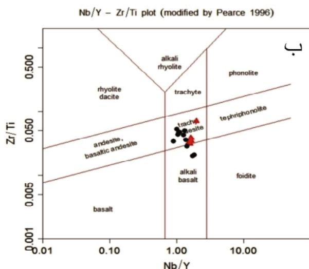
شکل ۳ الف) رده‌بندی سنگ‌های آذرین با استفاده از نمودار مجموعه‌ی قلیایی نسبت به سیلیس [۱۱]. شکل ۳ ب) رده‌بندی سنگ‌های منطقه‌ی مورد بررسی با استفاده از نمودار Nb/Y - Zr/Ti [۱۲]. نماد مثلث وجود سنگ‌های نفوذی و دایره توپر سنگ‌های آتشفشانی را نشان می‌دهند.
