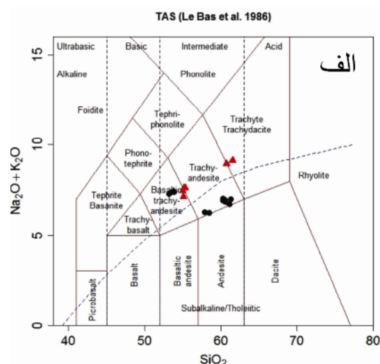
شکل ۳ الف) رده‌بندی سنگ‌های آذرین با استفاده از نمودار مجموعه‌ی قلیایی نسبت به سیلیس [۱۱]. شکل ۳ ب) رده‌بندی سنگ‌های منطقه‌ی مورد بررسی با استفاده از نمودار Nb/Y - Zr/Ti [۱۲]. نماد مثلث وجود سنگ‌های نفوذی و دایره توپر سنگ‌های آتشفشانی را نشان می‌دهند.
