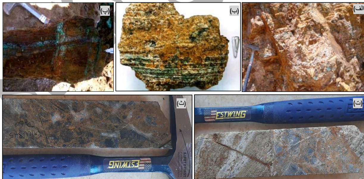
شکل ۷) تصاویری از بافت و ساخت لایه‌ای، لامینه‌ای، رگچه‌ای و برشی در کانسار قوزلو. الف) ساخت لایه‌ای در رخنمون ماده معدنی، تناوب لایه‌ای ماده معدنی (کالکوسیت کالکوپیریت و مالاکیت) و سیلیس در سنگ میزبان با ترکیب کربناتی (مرمری)، ب) نمونه دستی انتخاب شده از رخنمون ماده معدنی با بافت لامینه‌ای، پ) تشکیل کانه‌زایی مس به صورت مالاکیت با بافت رگچه‌ای، ت، ث) نمونه مغزه‌های حفاری با بافت برشی.
