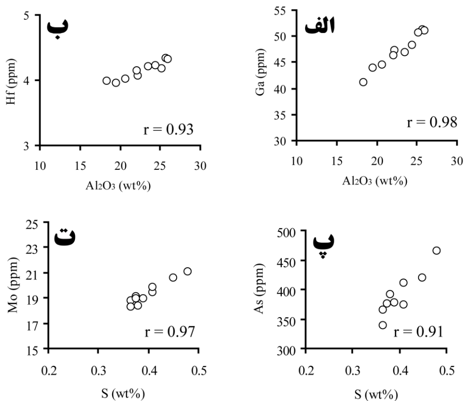
شکل ۸ نمودار دو متغیره \text{Al}_2\text{O}_3 -Ga (الف)، \text{Al}_2\text{O}_3 -Hf (ب)، S-As (پ) و S-Mo (ت) برای نمونه‌های مطالعه شده از پهنه دگرسانی آرژلیک منطقه شنین، غرب تاجیکستان.
