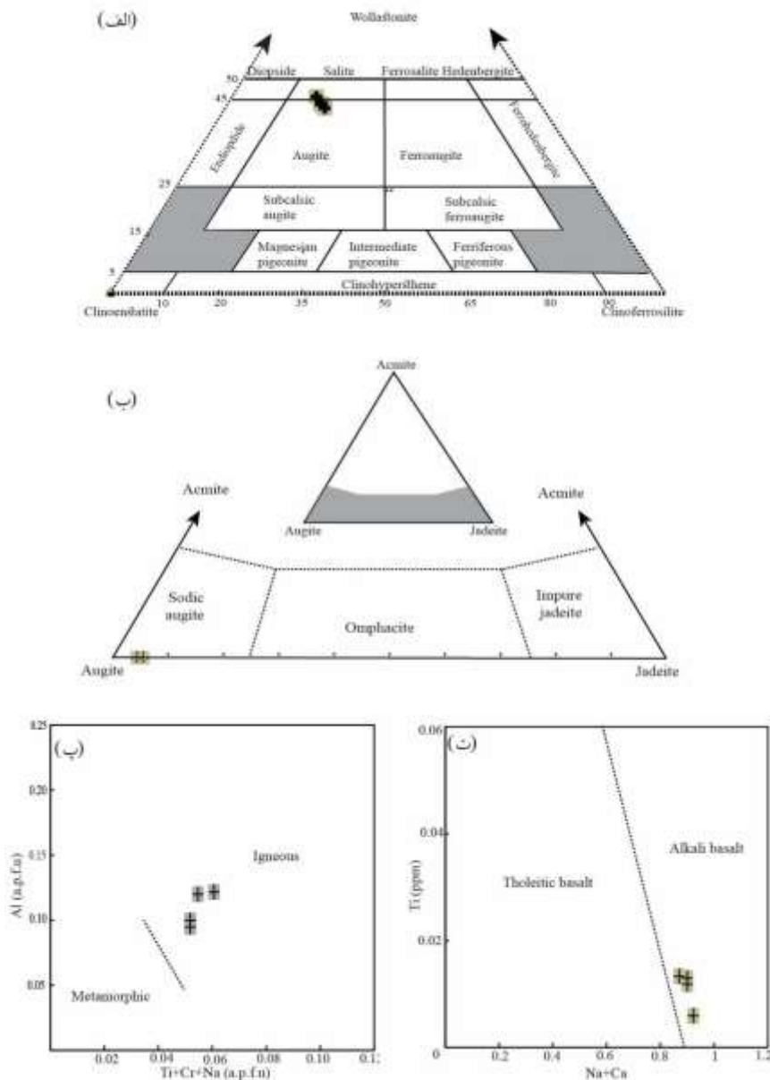
شکل ۶ موقعیت بلورهای کلینوپیروکسن توده متاگابرویی در (الف) نمودار Wo-Cen-Cfs [۱۰]، (ب) نمودار Acm-Aug-Jd [۱۱]، (پ) نمودار Al/Ti+Cr+Na ، تفکیک کننده پیروکسن‌های آذرین و دگرگون [۹] و (ت) نمودار Ti/Na+Ca ، تعیین کننده سری ماگمایی بر اساس شیمی پیروکسن [۱۲]. بر این اساس، بلورهای پیروکسن ماهیت آذرین و ترکیب اوزیتی دارد و از ماگمایی با ترکیب قلیایی شکل گرفته‌اند.
