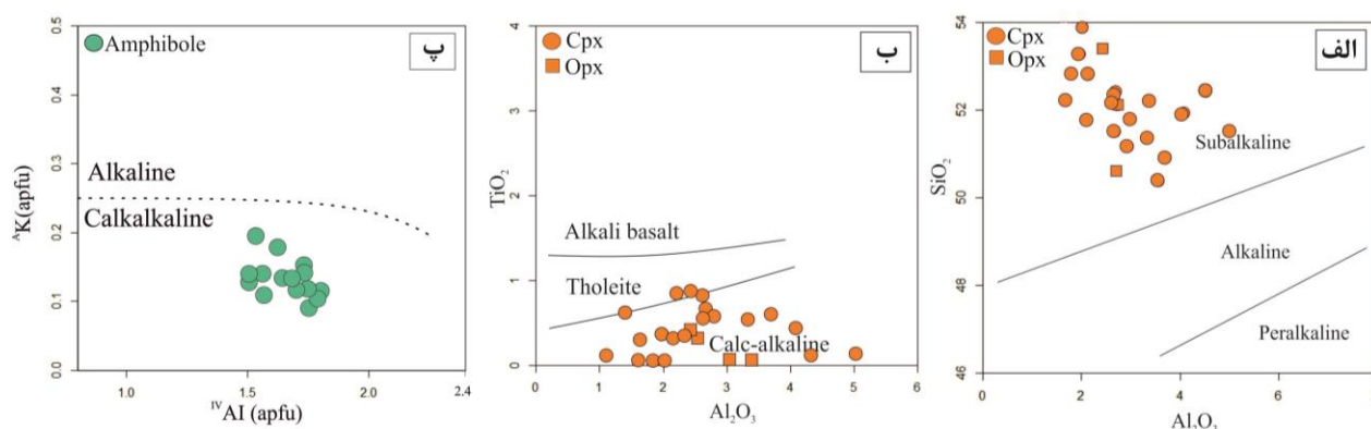
شکل ۹ الف موقعیت نمونه‌ها در نمودار Al_2O_3 نسبت به SiO_2 [۲۷]؛ ب) نمودار TiO_2 نسبت به Al_2O_3 که براساس آن نمونه‌ها ویژگی آهکی قلیایی دارند [۲]؛ پ) نمودار Al^{IV} نسبت به K^{IV} [۲۹] که ویژگی آهکی قلیایی آمفیبول‌های نمونه‌های مورد بررسی را نشان می‌دهد.
