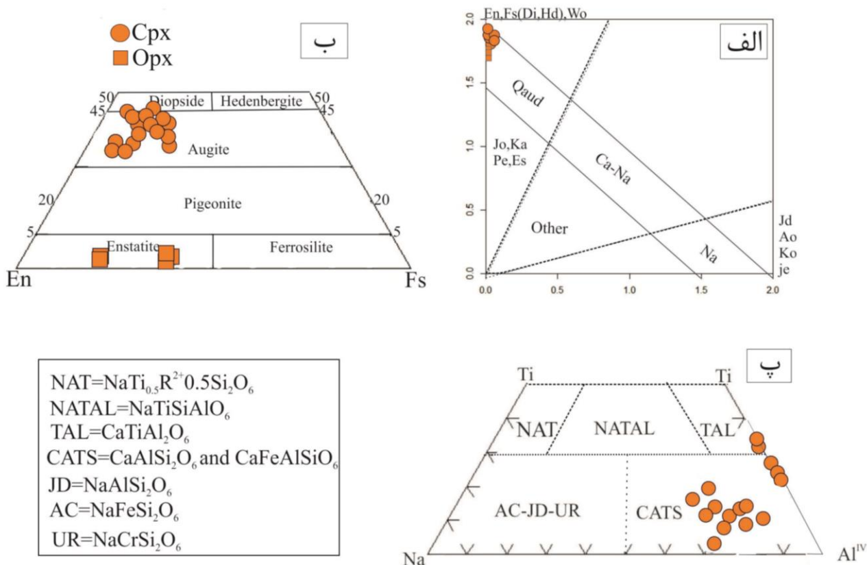
شکل ۷ الف نمودار رده‌بندی پیروکسن‌ها [۲۴]، که در آن پیروکسن‌های مورد بررسی در بخش آهن-منیزیم-کلسیم (Qaud) جایابی شده‌اند؛ ب) نمودار مثلثی Wo-En-Fs [۲۴] نشان می‌دهد که پیروکسن‌ها از نوع اوژیت و انستاتیت هستند؛ پ) نمودار مثلثی Ti-Na-Al IV [۲۵] که گویای ویژگی غنی از کلسیم بودن کلینوپیروکسن‌های مورد بررسی است.
