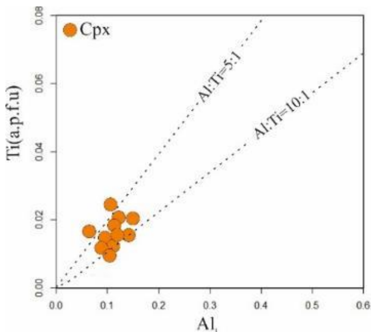
شکل ۸ نمودار موازنه نسبت Ti به Al I [۲۶] کلینوپیروکسن‌های مورد بررسی.
