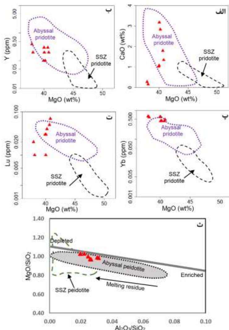
شکل ۱۰ موقعیت پریدوتیت‌های میزبان کرومیت قشلاق در نمودارهای، الف تا ت) تغییرات اکسید کلسیم و عناصر کمیاب (Yb و Lu، Y) نسبت به MgO. گستره‌های مربوط به پریدوتیت‌های مغاک و پهنه بالای فروران‌ش به ترتیب برگرفته از مراجع [۳۸، ۳۷] هستند. ث) موقعیت پریدوتیت‌های قشلاق در نمودار تغییرات MgO/SiO_2 نسبت به Al_2O_3/SiO_2 [۳۶].
