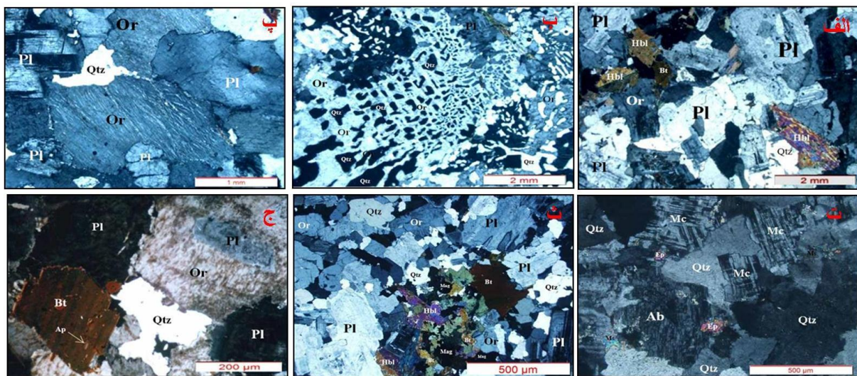
شکل ۴ الف) بافت دانه‌ای و هورنبلند اسکلتی و گردشده در توده مونزوگرانیت امین‌آباد، (در نور قطبیده متقاطع، Xpl)، ب) بافت گرافیکی در توده مونزوگرانیت امین‌آباد (Xpl)، پ) پرتیت رشته‌ای، همراه با کوارتز و پلاژیوکلاز در توده امین‌آباد، ت) بافت دانه‌ای همراه با درشت بلور پلاژیوکلاز با بافت صفحه شطرنجی در توده ارجنان، ث) هورنبلند و بیوتیت همراه با کانی‌های فلسی در ارجنان، ج) درشت بلورهای پلاژیوکلاز، کوارتز و بیوتیت در توده گرانیتوئیدی ارجنان.
