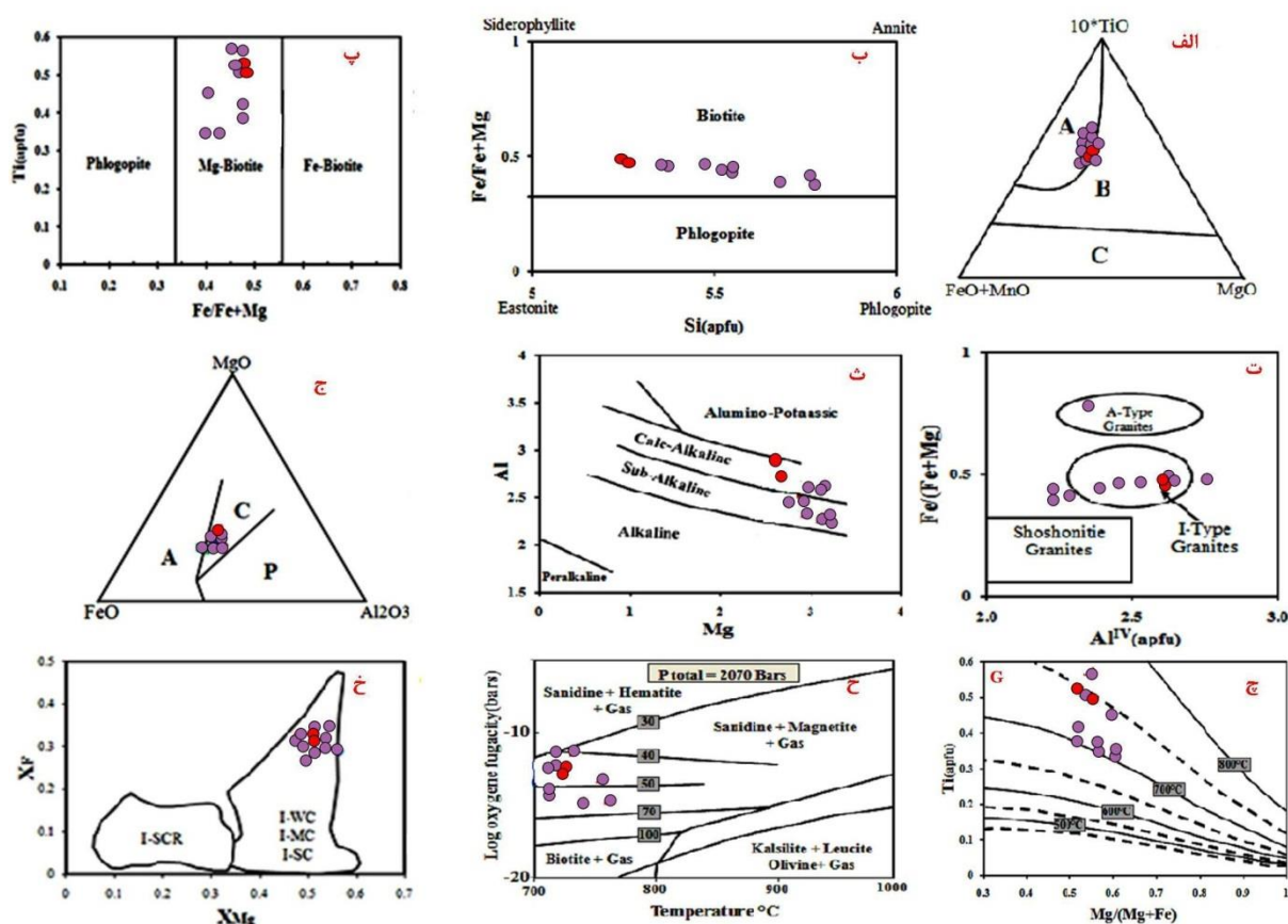
شکل ۸ الف) نمودار سه تایی تمایز انواع بیوتیت‌ها [۲۸]، ب) رده‌بندی شیمیایی میکاهای توده نفوذی مورد بررسی در نمودار مرجع [۳۳]، پ) نمودار مثلثی \text{MgO-FeO-Al}_2\text{O}_3 [۲۹] و جایگاه ترکیب شیمیایی بیوتیت‌ها، ت) نمودار درجه اشباع‌شدگی آلومینیم بیوتیت‌های مورد بررسی نسبت به سنگ میزبان [۳۴]، ث) نمایش نمونه‌های بیوتیت در نمودار تغییرات \text{Fe}/(\text{Fe}+\text{Mg}) نسبت به \text{Al}^{\text{IV}} [۳۲]، ج) نمودار مثلثی \text{FeO-MgO-Al}_2\text{O}_3 برای رده‌بندی نوع سری ماگمای گرانیتوئیدی، چ) نمودار تعیین دما با استفاده از مقدار تیتان بیوتیت‌ها [۳۵]، ح) جایابی نمونه‌ها در نمودار تغییرات \text{Log } f\text{O}_2 نسبت به دما [۱۸]، خ) جایابی نمونه‌های بیوتیت‌های هامانه در نمودارهای برآورد میزان آلودگی پوسته‌ای.
