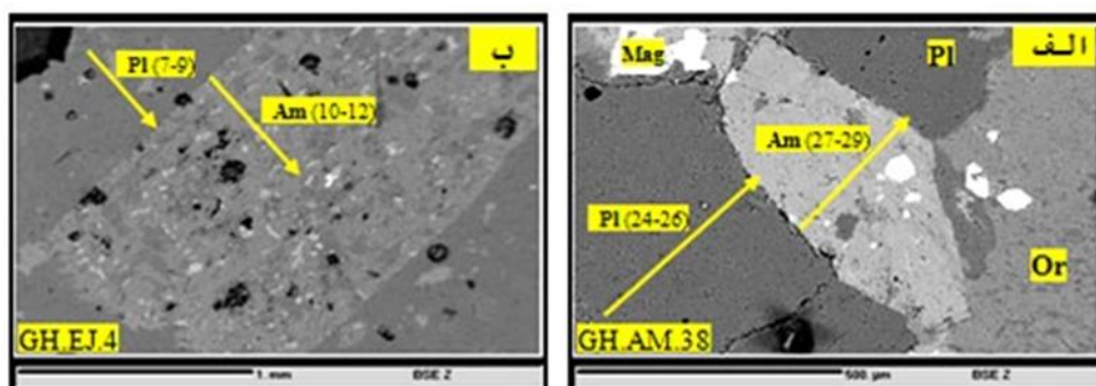
شکل ۵ تصاویر BSE از الف) آمفیبول شکل دار همزیست با پلاژیوکلاز، ارتوز، کوارتز و مگنتیت در مونزوگرنایت امین آباد، ب) آمفیبول با ترکیب منیزیهورنبلند و ترمولیت - اکتینولیت با ماکل کارلسباد و در تعادل با پلاژیوکلاز در گرانودیوریت ارجنان.
