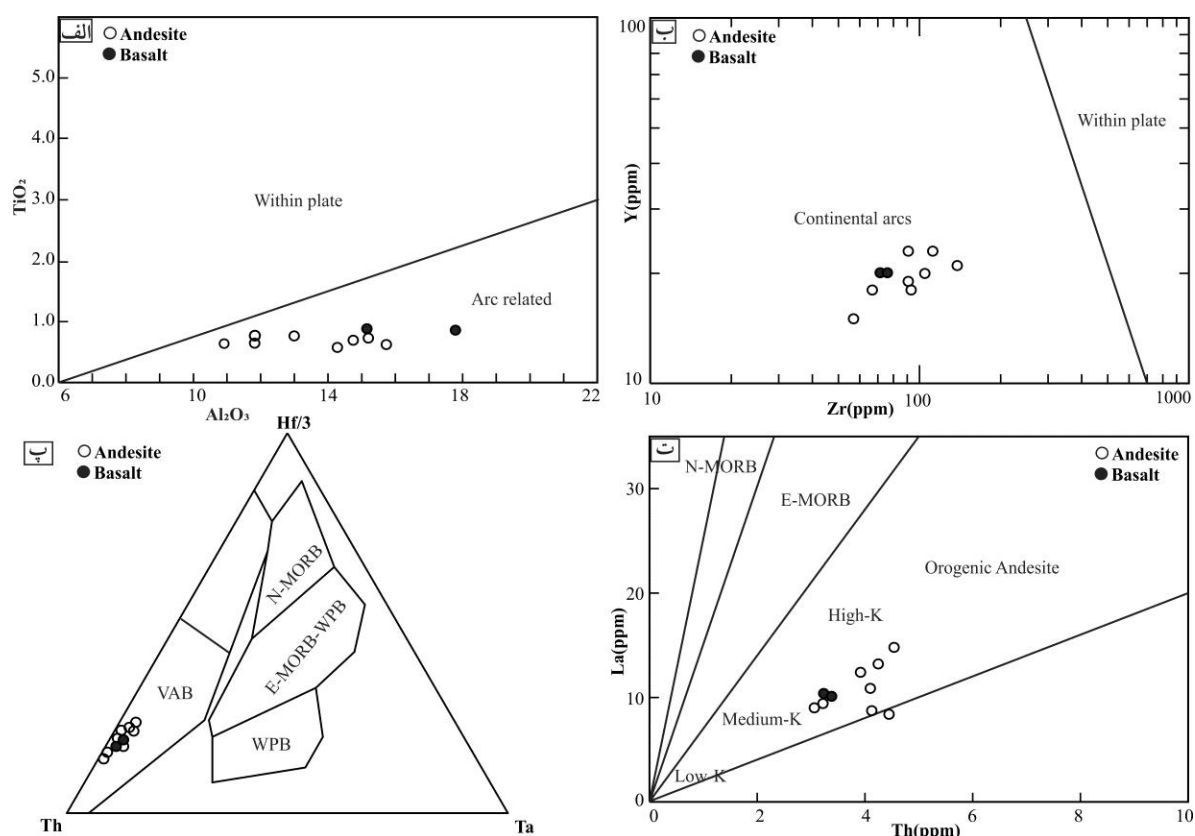
شکل ۸ نمودارهای زمین شیمیایی تعیین محیط زمین ساختی سنگ‌های آتشفشانی کوه بندسیاه (شمال غرب انارک): (الف) نمودار \text{TiO}_2 - \text{Al}_2\text{O}_3 برای نمونه‌های (الف) (ب) نمودار \text{Y} - \text{Zr} (ج) نمودار \text{Hf}/3 - \text{Th} - \text{Ta} (د) نمودار \text{La} - \text{Th} برای تفکیک مذب‌های در ارتباط با بازشدگی‌ها و مذب‌های تشکیل شده در محیط‌های کمان [۵۷]، (پ) نمودار مثلی برای تفکیک مذب‌های در ارتباط با بازشدگی‌ها و مذب‌های تشکیل شده در محیط‌های کمان [۵۷]، (ت) نمودار \text{La} - \text{Th} برای تفکیک آندزیت‌های کوهزایی از سایر آندزیت‌ها [۵۶].
