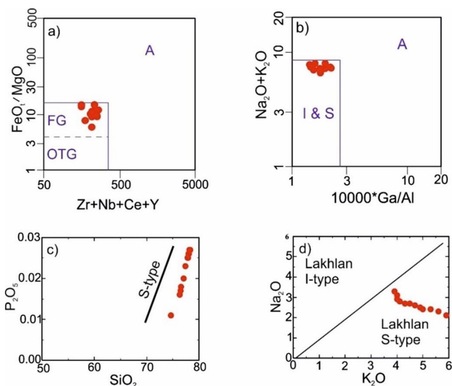
شکل ۱۴ نمودارهای تعیین کننده نوع گرانیتوئیدها: الف و ب) نمودارهای دوتایی \text{FeO}_t/\text{MgO} نسبت به \text{Zr+Nb+Ce+Y} و \text{Na}_2\text{O}+\text{K}_2\text{O} نسبت به \text{Ga/Al} [۲۸] برای تفکیک گرانیتوئیدهای نوع A از I و S و M، پ و ت) نمودارهای \text{P}_2\text{O}_5 نسبت به \text{SiO}_2 [۲۹] و \text{Na}_2\text{O} نسبت به \text{K}_2\text{O} [۳۰] برای تفکیک گرانیتوئیدهای نوع I از S.
