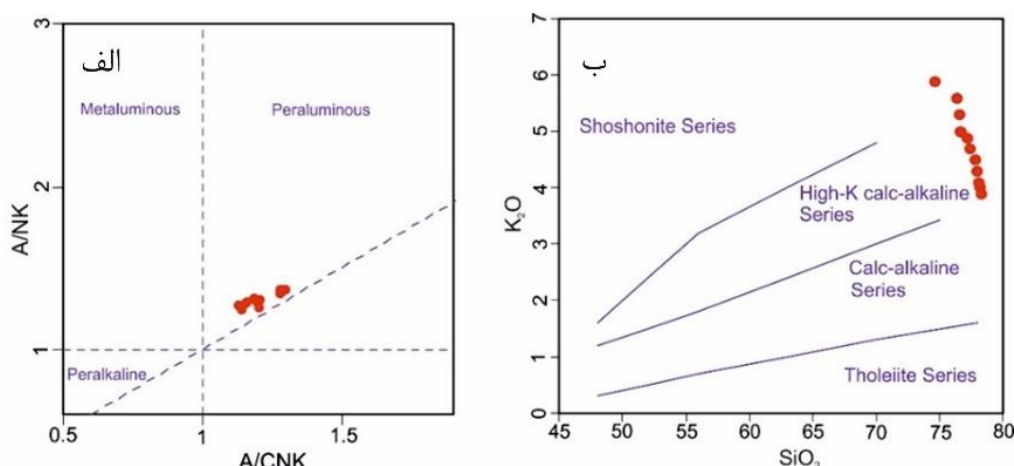
شکل ۱۱ الف) نمودار A/NK نسبت به A/CNK [۱۸]، برای تعیین اشباع‌شدگی از آلومینیم ماگما، ب) نمودار درصد وزنی K 2 O نسبت به SiO 2 [۱۹]، نمونه‌ها در گستره آهکی قلیایی پتاسیم بالا جای دارند.
