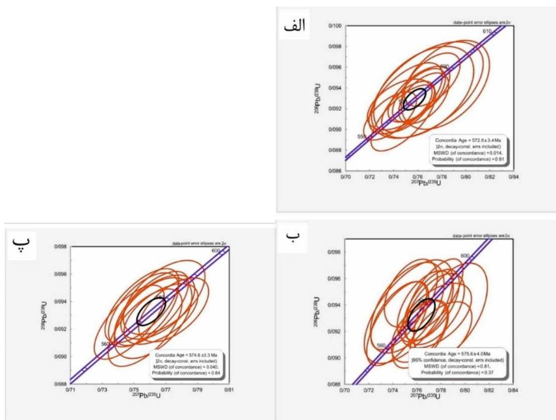
شکل ۹ نمودارهای سازوکار از داده‌های به‌دست‌آمده از سن‌سنجی با روش U-Pb زیرکن‌های سنگ‌های لوکوگرانیته مویه از الف) نمونه Mu-7D، ب) نمونه Mu-13D، پ) نمونه Mu-14D.
