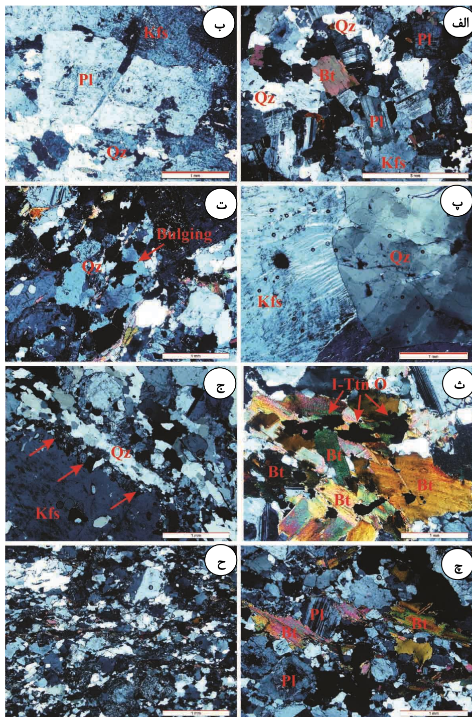
شکل ۴ تصاویر میکروسکوپی انواع ریزساخت‌ها در سنگ‌های توده گرانیتوئیدی گراغه در نور قطبیده متقاطع (XPL): الف) بافت ماگمایی که با بلورهای تخته‌ای شکل پلاژیوکلاز، کانی‌های سالم کوارتز و بیوتیت مشخص می‌شود. ب) بافت نیمه ماگمایی که در آن، پلاژیوکلاز شکسته شده و با کوارتز \pm فلدسپار پتاسیم پر شده است، پ) خاموشی صفحه شطرنجی کوارتز و بافت پرتیتی، ت) کوارتزهای دگرشکل شده با مرزهای دنداندار، ث) تیتانومگنتیت در بلورهای بیوتیت. ج) بافت میرمیکتی (به راستاهای پیکان‌ها دقت نمایید)، چ و ح) بیوتیت‌های دگرشکل شده که بصورت میکا ماهی در آمده‌اند. نشانه‌های اختصاری برگرفته از مرجع [۱۹] هستند.
