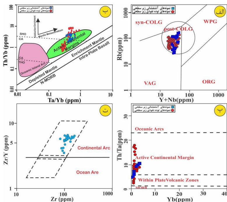
شکل ۶ نمودارهای تفکیک محیط زمین‌ساختی توده‌های نفوذی و واحدهای آتشفشانی گستره معدنی تازه‌کند، نمودار Rb نسبت به Y+Nb به (الف)، نمودار Th/Yb نسبت به Ta/Yb به (ب)، نمودار Th/Ta نسبت به Yb به (پ) و نمودار Zr/Y نسبت به Zr برای نمونه‌های آتشفشانی [۲۷].
