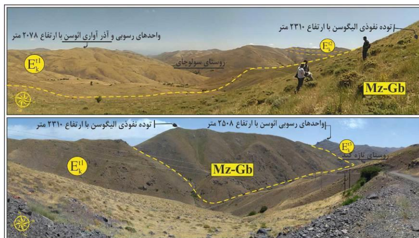
شکل ۲ تصاویر صحرایی از گستره معدنی تازه‌کند که توده‌های نفوذی با ترکیب سنگ‌شناسی مونزونیت تا گابرو به سن الیگومیوسن، واحدهای آتشفشانی- رسوبی آئوسن را قطع کرده‌اند.
