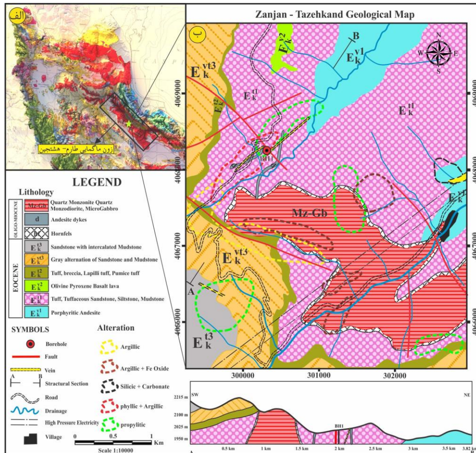
شکل ۱ الف) نقشه پهنه‌های ساختاری شمال غرب ایران و جایگاه کمر بند ماگمایی طارم- هشتجین [۱-۳]، ب) نقشه زمین‌شناسی با مقیاس ۱:۱۰۰۰۰ برای منطقه تازه‌کند به همراه برونزد پهنه‌های دگرسانی برگرفته از مرجع [۱۵].
