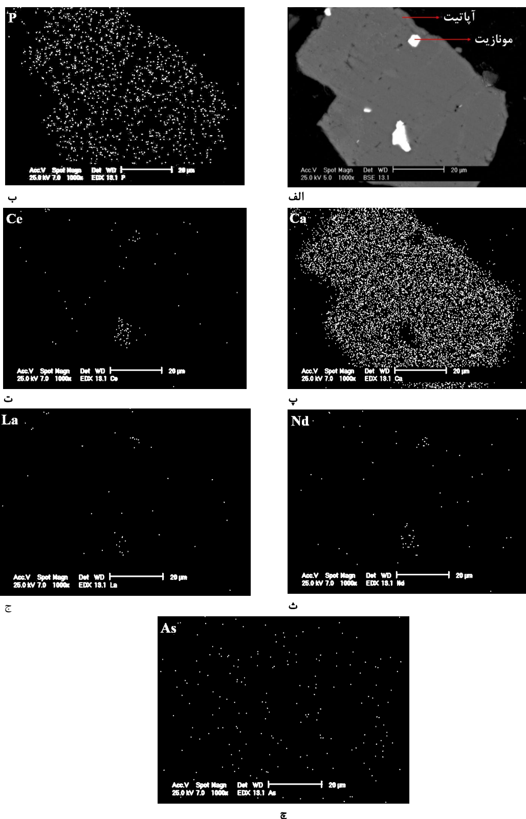
شکل ۴ نتایج بررسی با میکروسکوپ الکترونی: (الف) ذره‌هایی از کانی مونازیت درون آپاتیت، (ب) نقشه توزیع فسفر در شکل الف، (پ) نقشه توزیع کلسیم در شکل الف، (ت) نقشه توزیع سریم در شکل الف، (ث) نقشه توزیع نفودیمیموم در شکل الف، (ج) نقشه توزیع لانتانیم در شکل الف، (چ) نقشه توزیع آرسنیک در شکل الف.
