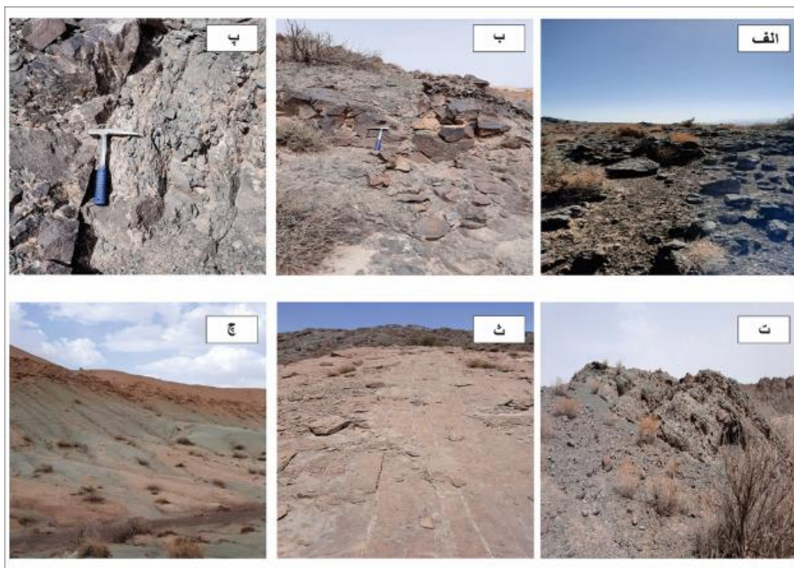
شکل ۴: تصاویری از واحدهای سنگی منطقه کلاته برق: (الف) واحد الیوین بازالت (دید به سمت شمال غربی)، (ب) واحد آندزیتی تیره رنگ (دید به سمت شمال غربی)، (پ) واحد هورنبلند پیروکسن دیوریت، (ت) واحد کنگلومرای (دید به سمت جنوب غربی)، (ث) واحد سنگ‌آهک نومولیتی همراه با رگچه‌های کلسیتی، (چ) واحد مارن.
