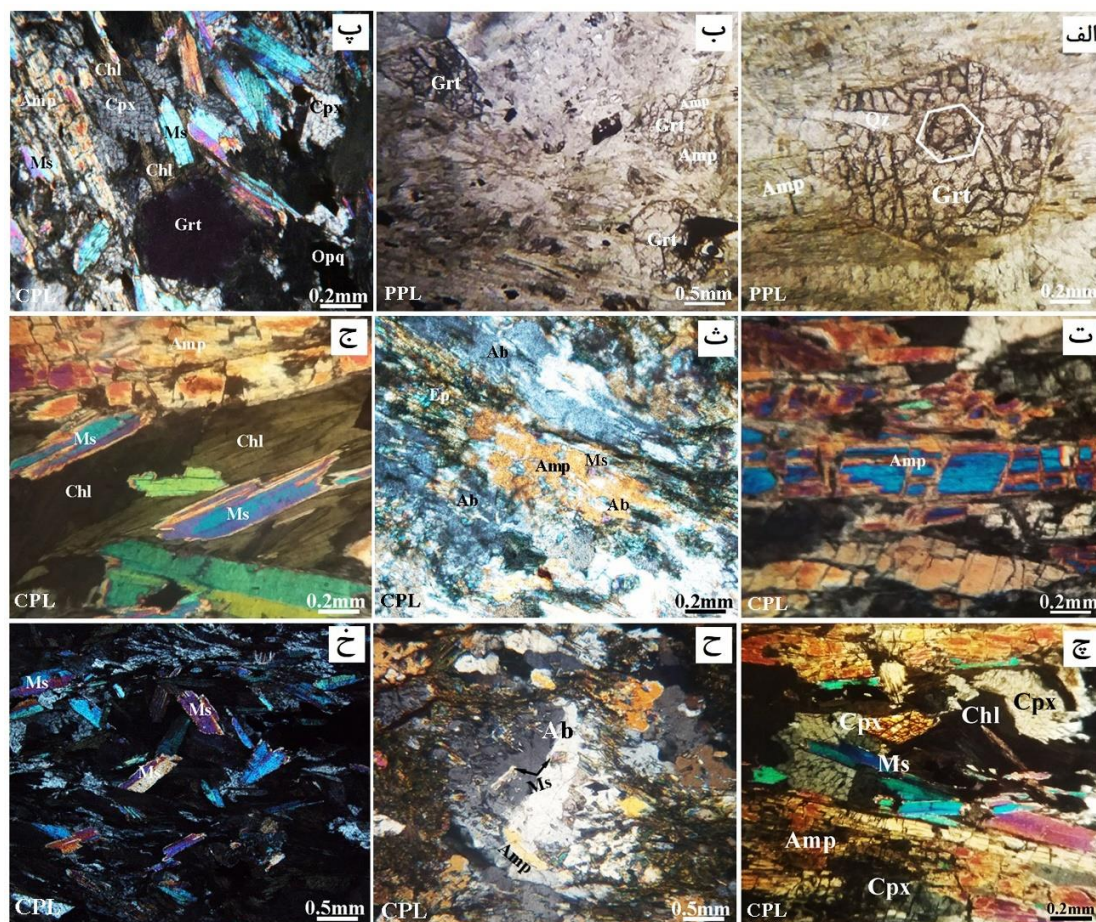
شکل ۲ تصاویر میکروسکوپی از کانی‌های تشکیل‌دهنده سنگ اکلوزیتی منطقه ویسدار. الف) گارنت دارای منطقه‌بندی با میانبرهای کوارتز، ب) گارنت با میانبرهای آمفیبول و کوارتز، پ) گارنت بدون میانبر، ت) آمفیبول موجود در شیشه‌توارگی با ساختار منطقه‌بندی، در مرکز ترکیب گلوکوفانی و در لبه ترکیب اکتینولیتی دارد، ث) آمفیبول غربالی با میانبرهایی از مسکویت و آل بیت همچنین کانی‌های اپیدوت و آل بیت در لبه فشارشی، ج) مرز واکنشی شکفته بلور آمفیبول با کانی‌های کلریت و مسکویت، چ) کلینوپیروکسن‌های دگرشکفت و نیمه خودشکفت با تبدیل‌شدگی به کلریت، مسکویت و آمفیبول، ح) شکفته بلور آل بیت با میانبرهایی از آمفیبول و میکای سفید و خ) شکفته بلورهای میکای سفید با جهت‌گیری مایل نسبت به شیشه‌توارگی.
