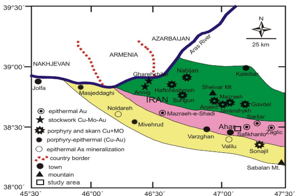
شکل ۱ توزیع پهنه‌های فلززایی و کانه‌زایی مختلف در کمربند سنوزوئیک اهر-ارسباران در شمال‌غرب ایران، برگرفته از مرجع [۱] با کمی تغییرات.
