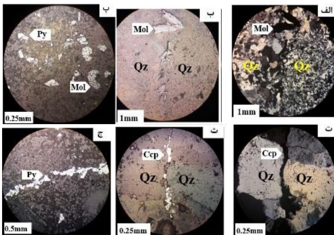
شکل ۴ تصاویر میکروسکوپی کان‌های فلزی در کانسار شله‌بران شامل، الف) حضور مولیبدنیت (Mol) به صورت رگچه‌ای درون بلورهای کوارتز (Qz) در نور عبوری (XPL، ب) تصویر الف در PPL، پ) حضور پیریت (Py) و مولیبدنیت (Mol) بصورت افشان در توده‌های نفوذی (گرانودیوریت) در نور عبوری (XPL، ت) حضور کالکوپیریت (Ccp) در رگه-رگچه‌های کوارتز-سولفیدی در نور عبوری (XPL، ث) تصویر ت در PPL و ج) حضور پیریت (Py) در رگه-رگچه‌های کوارتز-سولفیدی (در PPL). نشانه‌های اختصاری کانی‌ها برگرفته از مرجع [۳۰] هستند.
