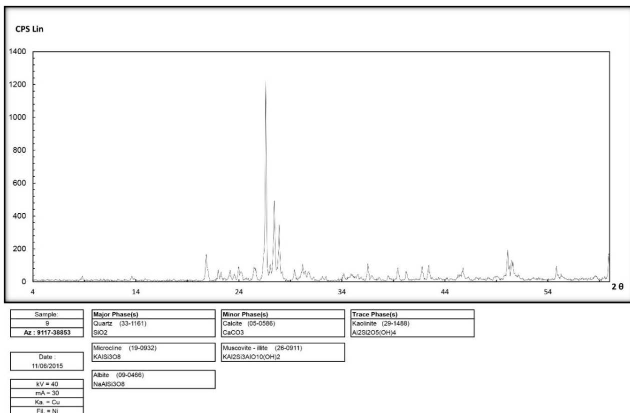
شکل ۷ طیف XRD وابسته به یکی از نمونه‌های ناحیه مسترون و حضور کوارتز، میکروکلین و آلbite به عنوان کانی اصلی، کلسیت و موسکوویت به عنوان کانی فرعی و کائولینیت به عنوان کانی جزئی.
