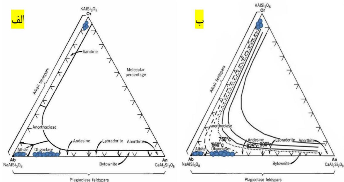
شکل ۸ الف) رده بندی پلاژیوکلازها براساس ترکیب شیمیایی [۳۳]، ب) نمودار آلbite-آنورتیت-ارتوز [۳۴، ۳۵] و قرارگیری نمونه‌ها در گستره دمایی ۵۵۰ تا ۶۰۰°C.
