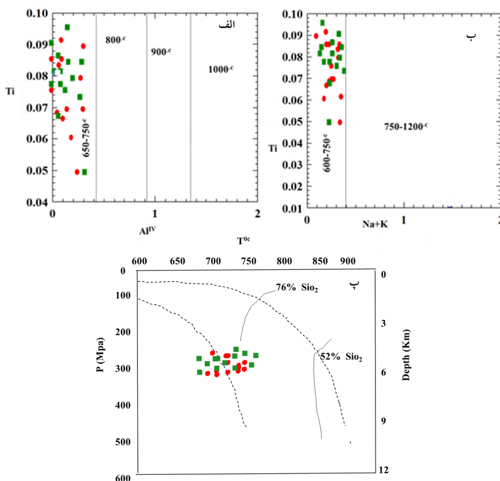
شکل ۶ الف: نمودار مقدار Ti نسبت به \text{Al}^{\text{IV}} [۲۲] برای تعیین دمای تشکیل آمفیبول‌ها، ب) نمودار Ti نسبت به \text{Na}+\text{K} [۵۹]، پ: جایابی نمونه‌های مورد بررسی منطقه در نمودار عمق، فشار و دما [۵۸].
