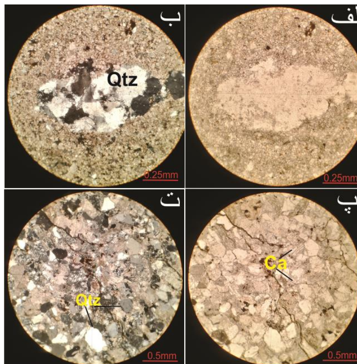
شکل ۵ تصویر میکروسکوپی الف وب) ماسه سنگی تیره (در نور قطبیده صفحه‌ای، ppl) گری وک؛ پ و ت) ماسه سنگ خرده سنگی (در نور قطبیده متقاطع، xpl): کوارتز، Qtz؛ کلریت، Clt؛ اکسید آهن، Fe-oxide؛ کربنات و Rf: خرده سنگ [۱۳].
