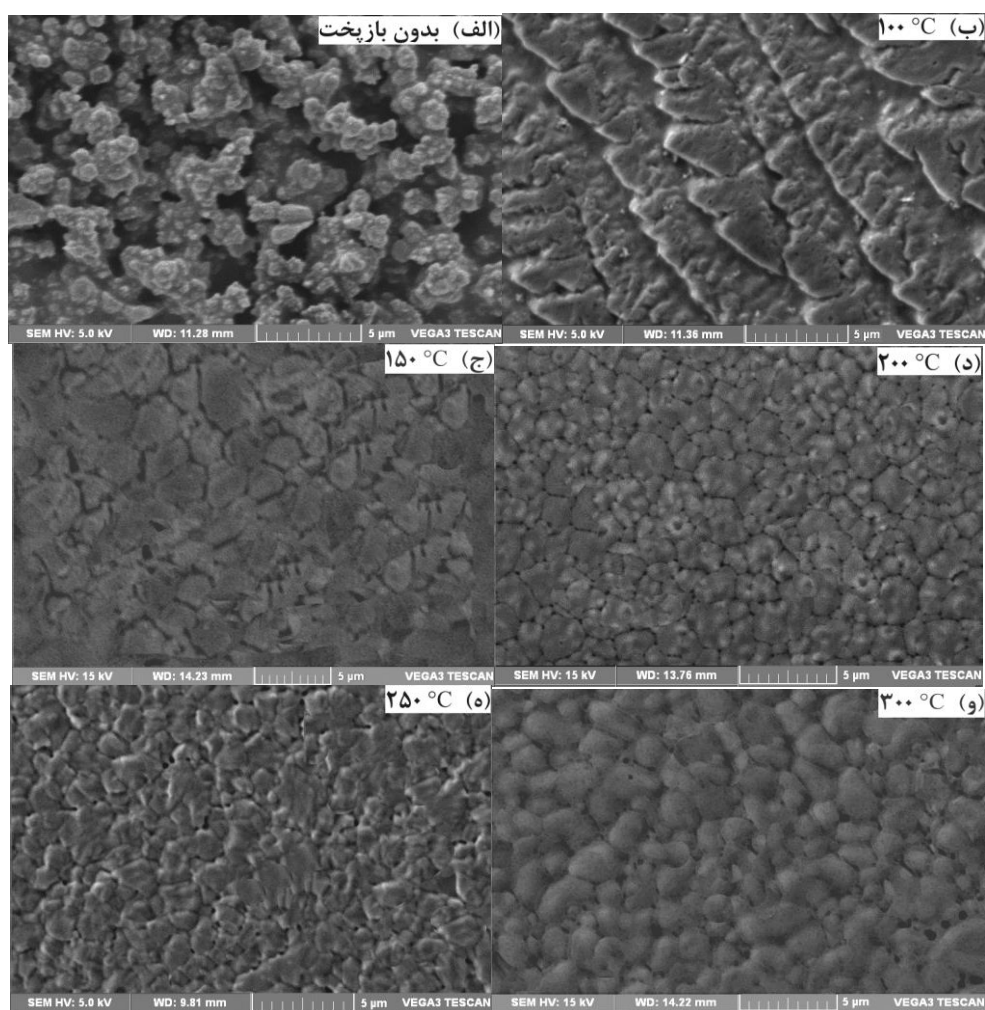
شکل ۵ تصاویر میکروسکوپ الکترونی روبشی لایه نازک پروسکایت \text{Cs}_2\text{AgBiI}_6 بازپخت‌شده در دمای مختلف.
