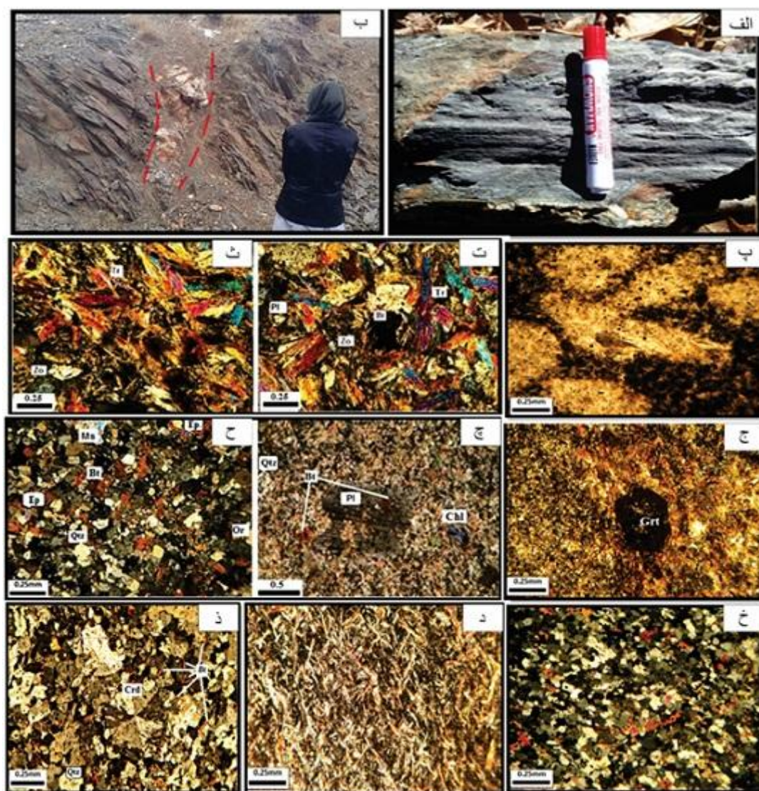
شکل ۳. (الف) تصویر ماکروسکوپی از ترمولیتیت. (ب) تصویر صحرایی از رگه کوارتزی نفوذ کرده در شیست‌ها در غرب وهنان، دید به سمت شمال غرب. (پ) تصویر میکروسکوپی از شیست لکه‌ای در نور قطبیده صفحه‌ای (PPL). (ت، ث) تصویر میکروسکوپی از ترمولیت در نور قطبیده متقاطع (XPL). (ج) تصویر میکروسکوپی از بافت شکفته بلوری که طی دگرگونی در یک زمینه دانه ریز رشد کرده است. (چ) تصویر میکروسکوپی از میکا هورنفلس. (ح، خ) تصویر بافت دانه شکفتی در نور XPL که این بافت ناشی از رخداد باز تبلور در یک سنگ و یا رسوب‌های از پیش موجود است. (د) تصویر میکروسکوپی از بافت نخ شکفتی در نور XPL. (ذ) تصویر میکروسکوپی از کردیریت هورنفلس با ماکل ساعت شنی در نور XPL.
