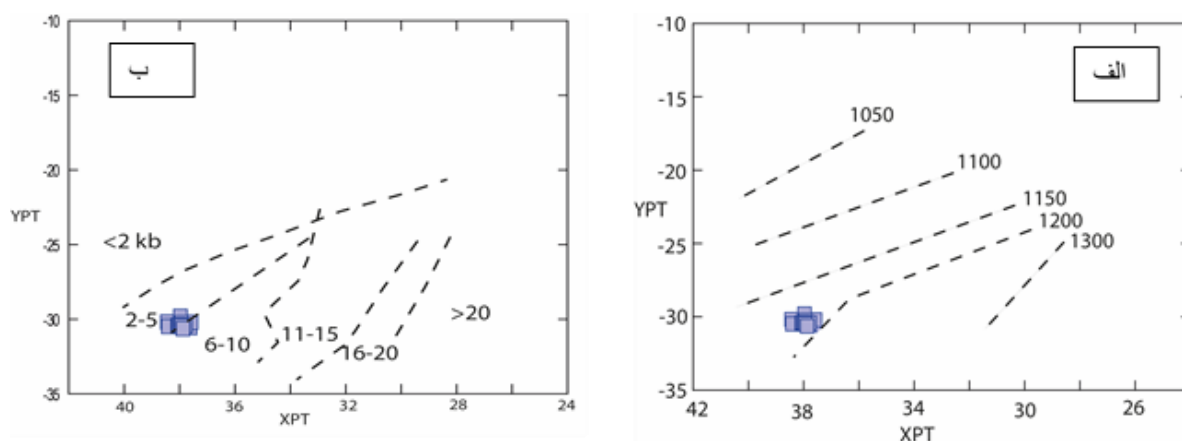
شکل ۱۲ الف و ب- نمودارهای Y_{PT} نسبت به X_{PT} [۲۹] برای دما-فشارسنجی سنگ‌های گابرویی مورد بررسی برپایه شیمی کلینوپیروکسن.
