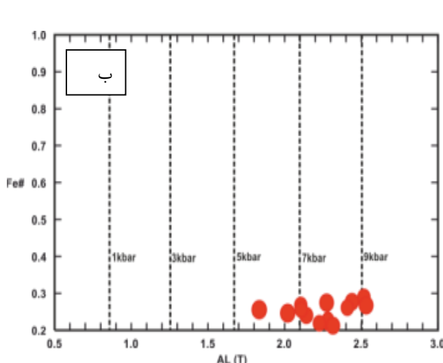
شکل ۱۳ همناهای Al_2O_3 و TiO_2 کلسیم آمفیبول‌ها براساس درصد وزنی به عنوان تابعی برای تعیین فشار و دما [۴۰] و موقعیت نمونه‌های مورد بررسی بر روی آن. ب- نمودار Fe/(Fe+Mg) نسبت به Al^{total} [۲۱] برای تعیین فشار تبلور آمفیبول‌های گابروهای مورد بررسی شترکوه.
