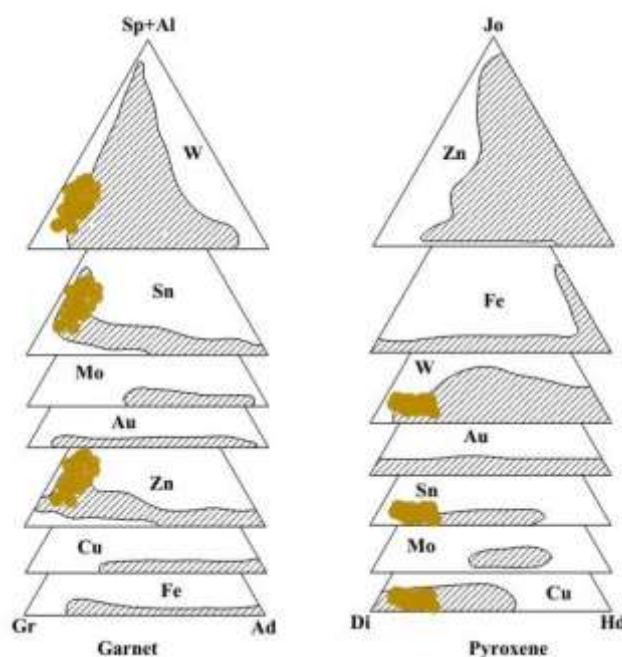
شکل ۸ مثلث‌های ترکیب‌های اعضای پایانی گارنت و پیروکسن در ارتباط با انواع اسکارن و احتمال کانه‌زایی مربوط به آنها [۳۳] (Ad: آندرادیت، Di: دیوپسید، Gr: گروسولاریت، Hd: هدنبرگیت، Jo: جوهانسنیت، پیرالسپیت = پیروپ + آلماندین + اسپسارتین).
