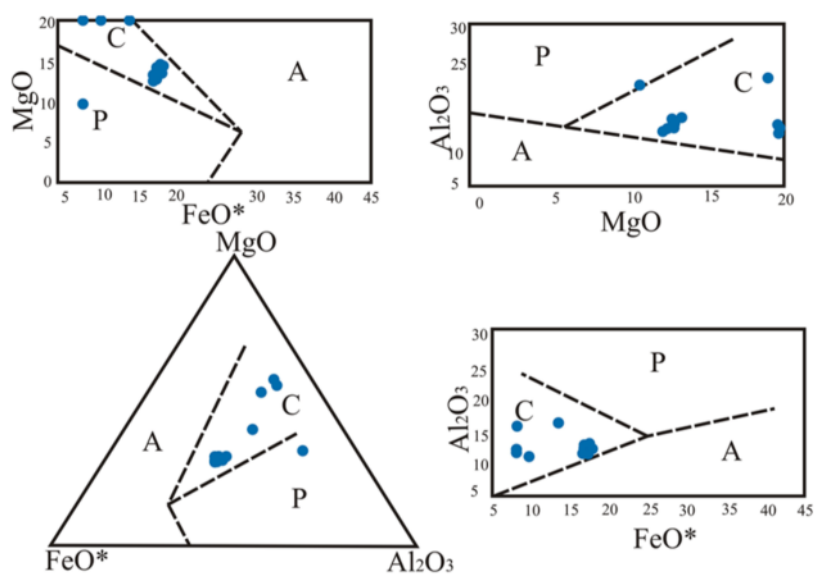
شکل ۱۶ تعیین سری ماگمایی بر پایه شیمی بیوتیت [۳۸]. A: قلیایی؛ C: آهکی قلیایی؛ P: پرآلومین.
