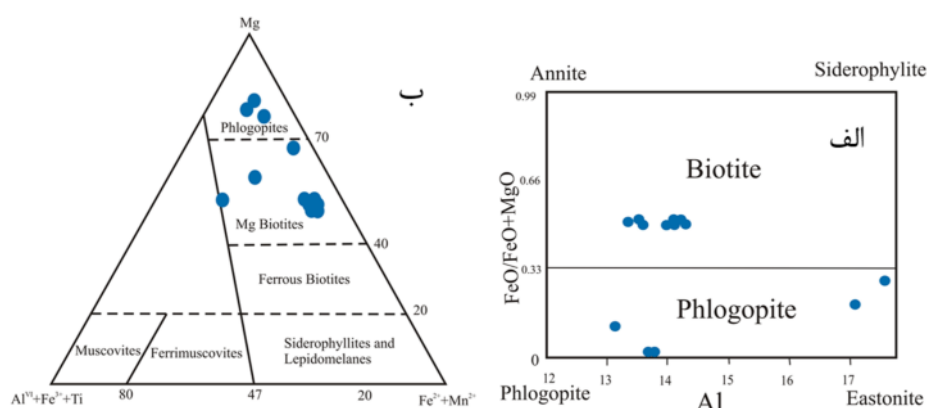
شکل ۱۴ الف) بررسی میکاهای آهن و منیزیم‌دار در نمودار چار قطبی [۳۵] و ب) براساس نمودار مرجع [۳۶] بیوتیت‌ها از نوع غنی از منیزیم هستند.
