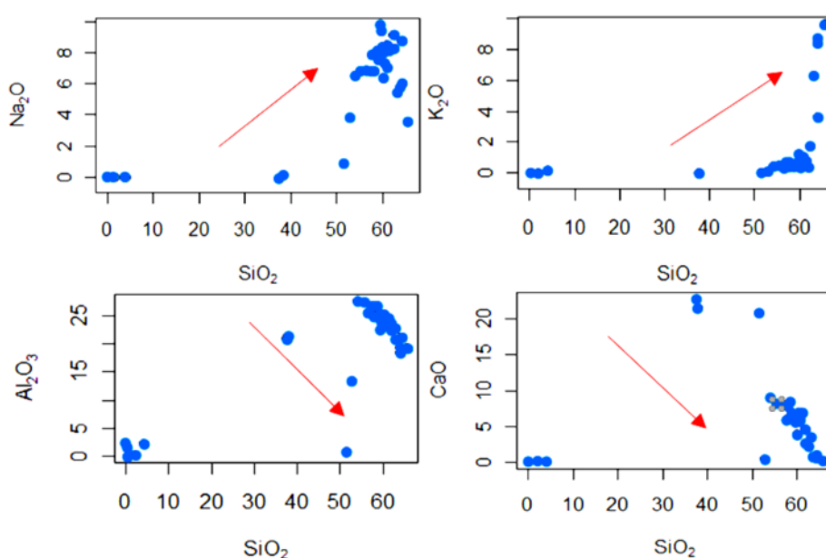
شکل ۶ تغییرات اکسید عناصر اصلی نسبت به SiO 2 .
