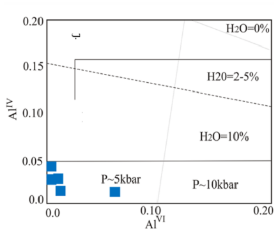
شکل ۱۰ الف) برآورد گریزندگی اکسیژن ماگما با استفاده از پیروکسن‌ها [۲۵]. ب) توزیع Al در جایگاه‌های چاروچی و هشت وجهی در کلینوپیروکسن‌ها به تناسب فشار و مقدار آب ماگما [۲۷].
