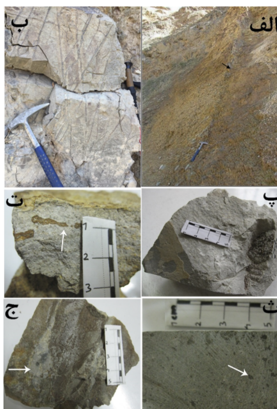
شکل ۵ تصاویر شکل‌های کانه‌سازی در منطقه مورد بررسی: (الف) رگه سیلیسی (پیکان) در واحد توف ائوسن (ب) دسته رگچه‌های سیلیسی در شیشه‌های ریولیتی شده (پ) رگچه اغلب پیریتی در نمونه توف با دگرسانی سریسیتی-آرژیلیکی (ت) افشان-لایه سولفیدی (اغلب پیریت) و اکسیدهای آهن (مگنتیت و هماتیت) همراه با اکسی-هیدروکسیدهای آهن با رنگ مایل به قهوه‌ای (برآمده از دگرسانی ثانویه). (ث) افشانه‌هایی از کانی‌سازی سولفیدی (پیریت، کالکوپیریت، گالن، اسفالریت، کوولیت و کالکوسیت) در نمونه توف با ترکیب حدواسط و با دگرسانی سریسیتی-آرژیلیکی (کانه‌ها با پیکان نشان داده شده‌اند) (ج) کانی‌سازی سولفیدی (پیکان) همراه رگچه سیلیسی در نمونه شیشه ریولیتی شده.
