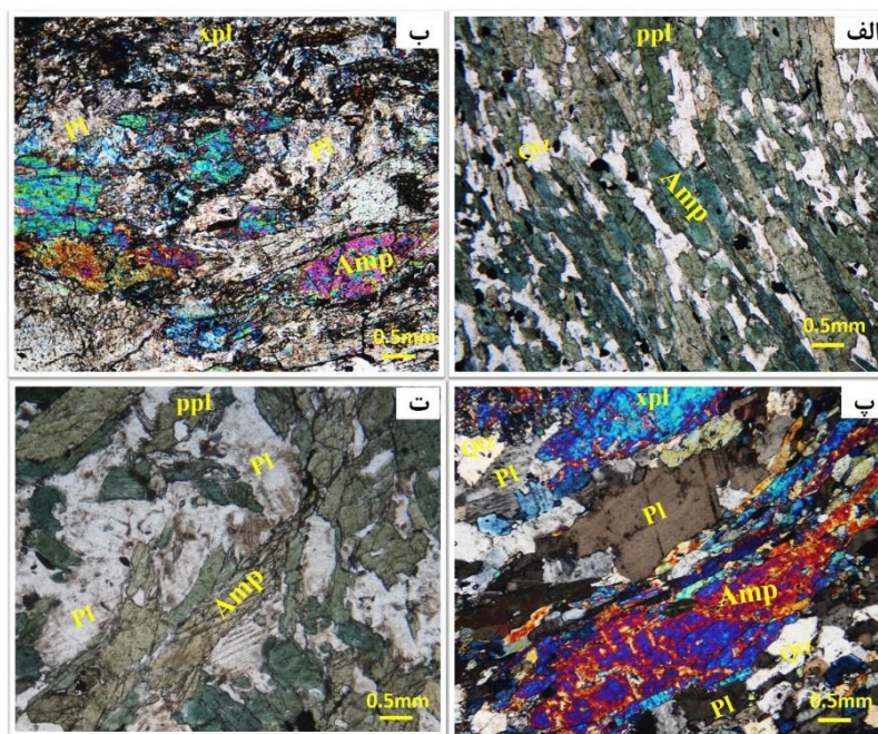
شکل ۵ تصاویر میکروسکوپی از آمفیبولیت‌ها: الف) تورق کنگره‌ای در آمفیبولیت‌های با چند رنگی سبز-آبی؛ ب) بافت نخ شکفتی، پ) تورق گنیسی و ت) پلاژیوکلازهای تقریباً دگرسان در آمفیبولیت، [آمفیبول (Amp)، پلاژیوکلاز (Pl)، گارنت (Gr)، کوآرتز (Qtz)، کلریت (Chl)].
