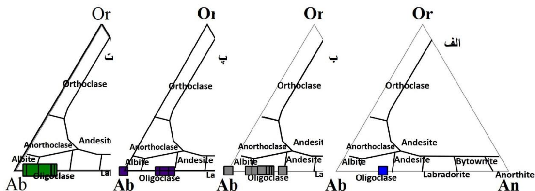
شکل ۷ الف، ب، ت) ترکیب فلدسپات در آمفیبولیت؛ (پ) ترکیب فلدسپات در اپیدوت آمفیبولیت [۲۵].
