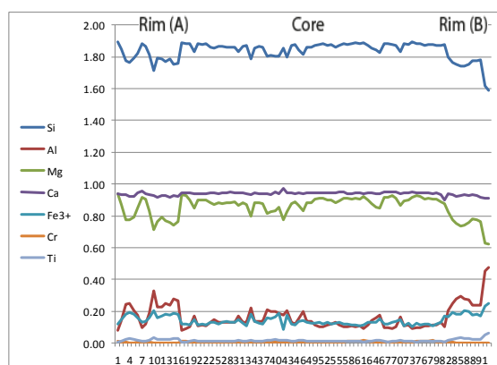
شکل ۴ روند توزیع عناصر در لبه A- مرکز- لبه B کلینوپروکسن. عنصر Ca و Fe 3+ از مرکز کانی به سمت هر دو لبه کانی، روند بدون تغییری نشان می‌دهند. عناصر Si و Mg از مرکز کانی به سمت هر دو لبه کانی روند کاهشی دارند.
