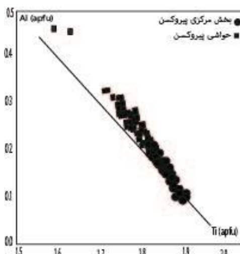
شکل ۷ نمودار Ti نسبت به Al [۲۹]. خط اشباع شدگی سیلیس و آلومینیوم در جایگاه چاروچی رسم شده است. قرارگیری نمونه‌های پیروکسن در بالای خط اشباع شدگی نشان دهنده مقادیر آلومینیوم است که پس از پر کردن جایگاه چاروچی، وارد جایگاه هشتوچی پیروکسن شده اند.
