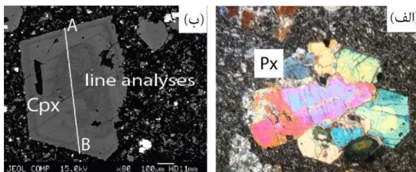
شکل ۳ (الف) تصاویر میکروسکوپی از سنگ‌های پیروکسن فیریک بازالت با بافت گلوپورفیری و بافت منطقه بندی کلینوپروکسن در نور قطبیده متقاطع، (XPL) در خمیره دگرسان شده، (ب) تصویر BSE از منطقه بندی پیروکسن‌ها، علائم بکار رفته برگرفته از مرجع [۱۷] هستند.
