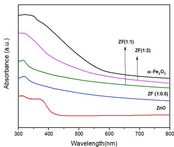
شکل ۴ طیف‌های جذب نمونه‌های ZnO، \alpha\text{-Fe}_2\text{O}_3 و نانوکامپوزیت‌های با درصد‌های وزنی مختلف \text{ZnO/Fe}_2\text{O}_3 .
