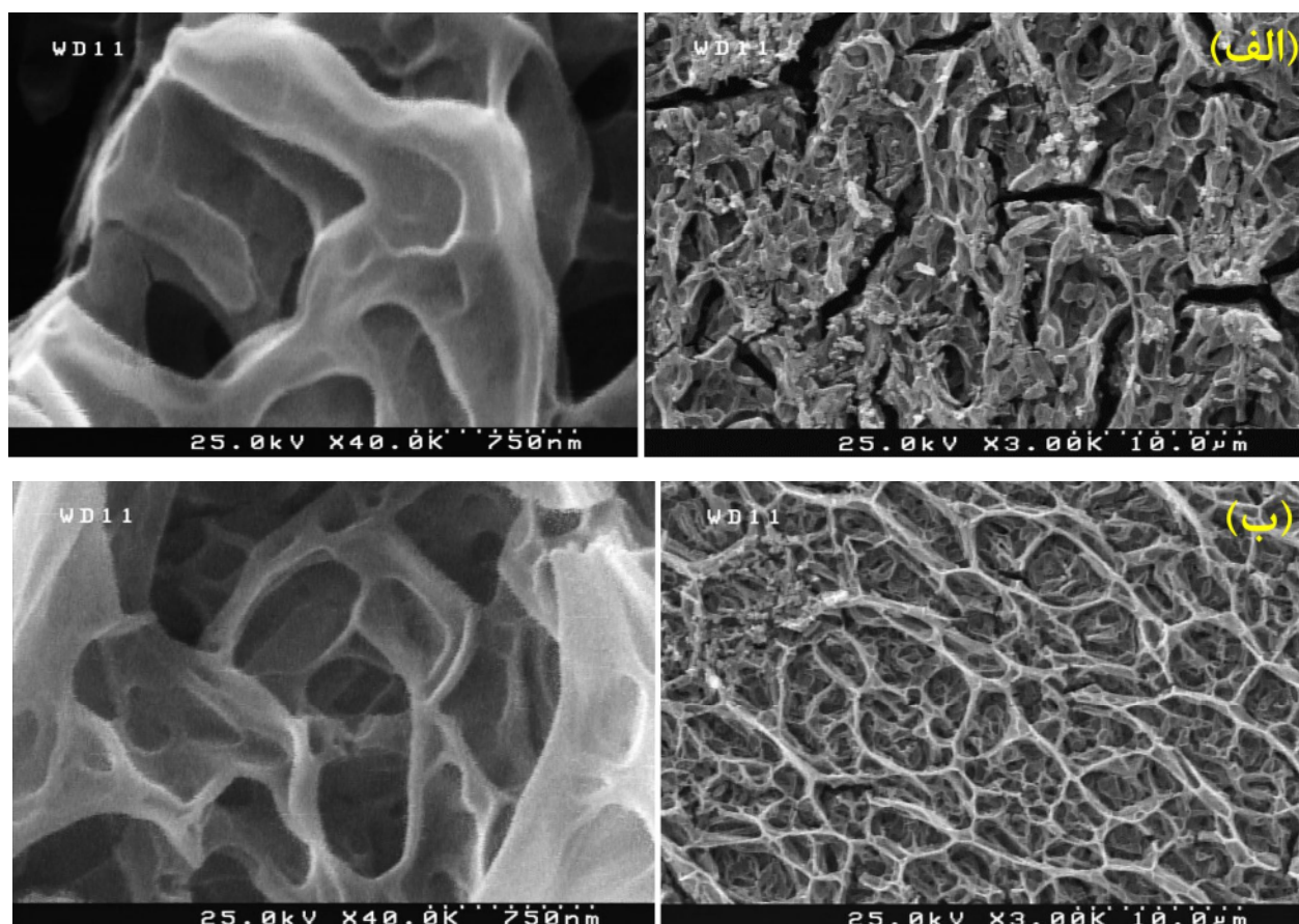
شکل ۵ تصاویر FESEM نمونه‌های سنتز شده با حجم محلول اولیه ۲۰۰ mL در حالت غیرپالسی (الف) زیرلایه FTO و (ب) زیرلایه شیشه در دو مقیاس 10\text{ }\mu\text{m} و 750\text{ nm}
