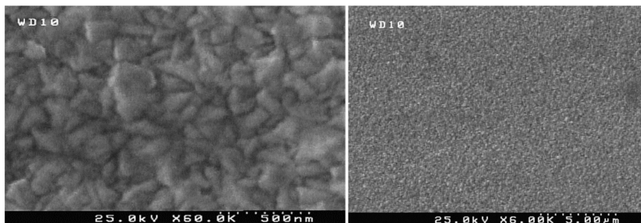
شکل ۴ ریخت‌شناسی سطح نمونه رسانای شفاف در نقش فوتون‌ها در مقیاس‌های 500\text{ nm} و 5\text{ }\mu\text{m} .
